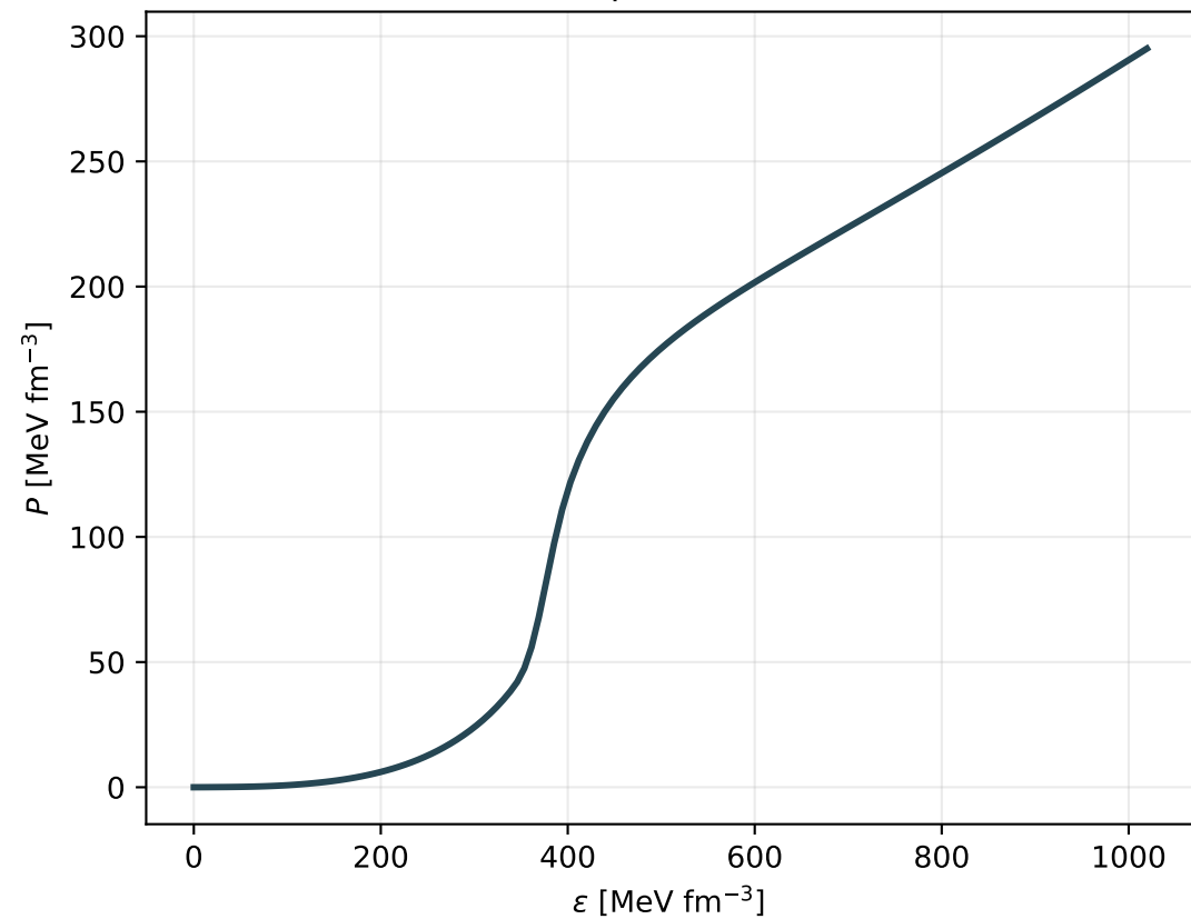
Beta-Equilibrium EOS
