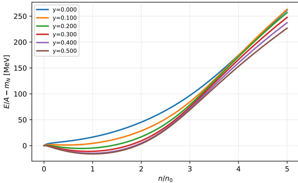
E/A - m_N
