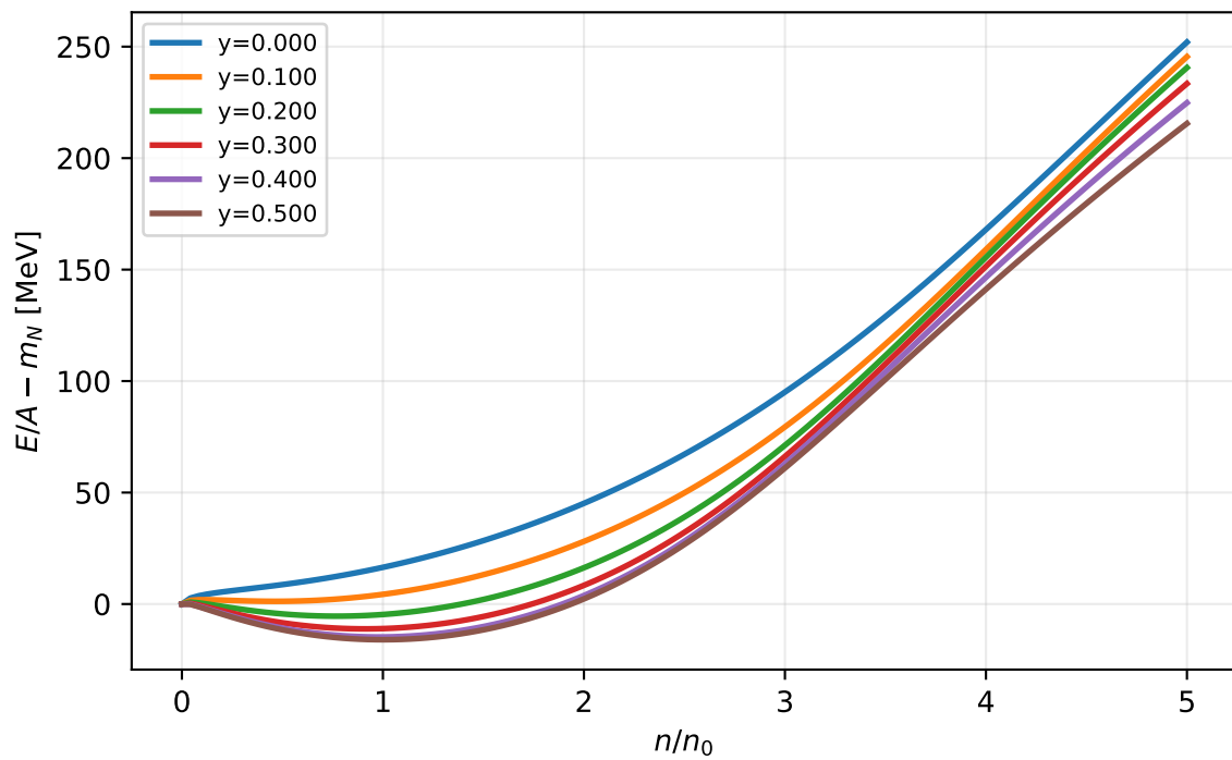
E/A - m_N
