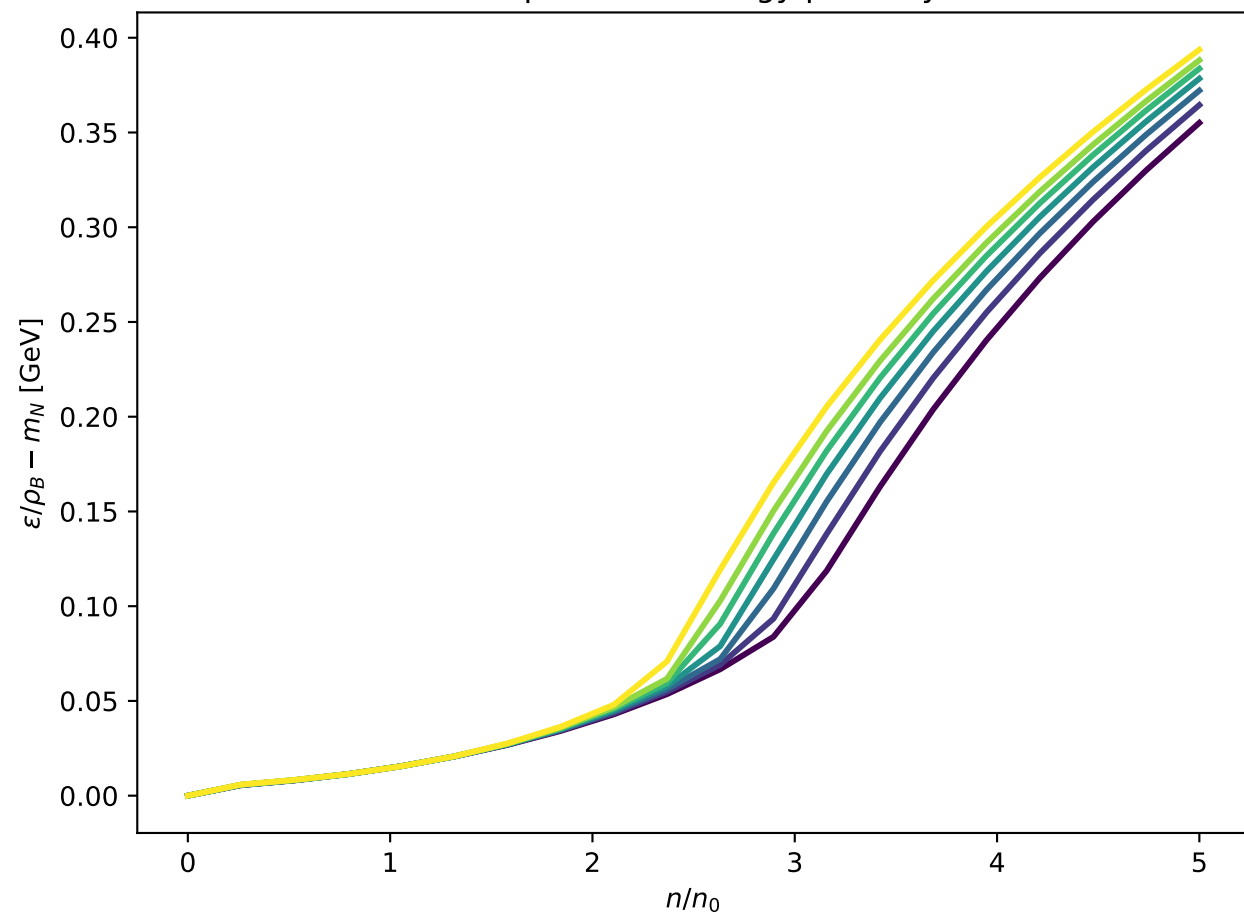
Beta-equilibrium energy per baryon
