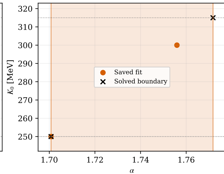
Clausius-TVM
