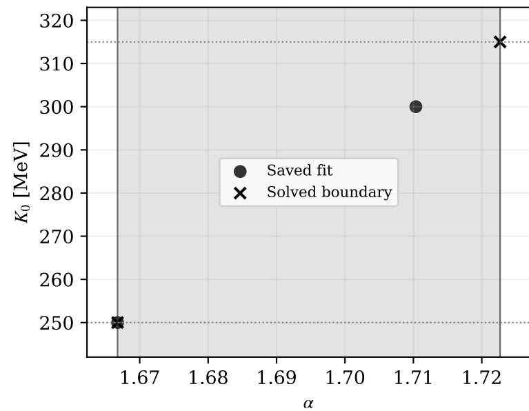
Clausius-VDW
