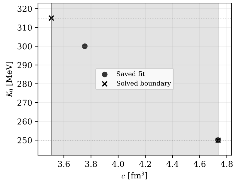
Clausius-VDW
