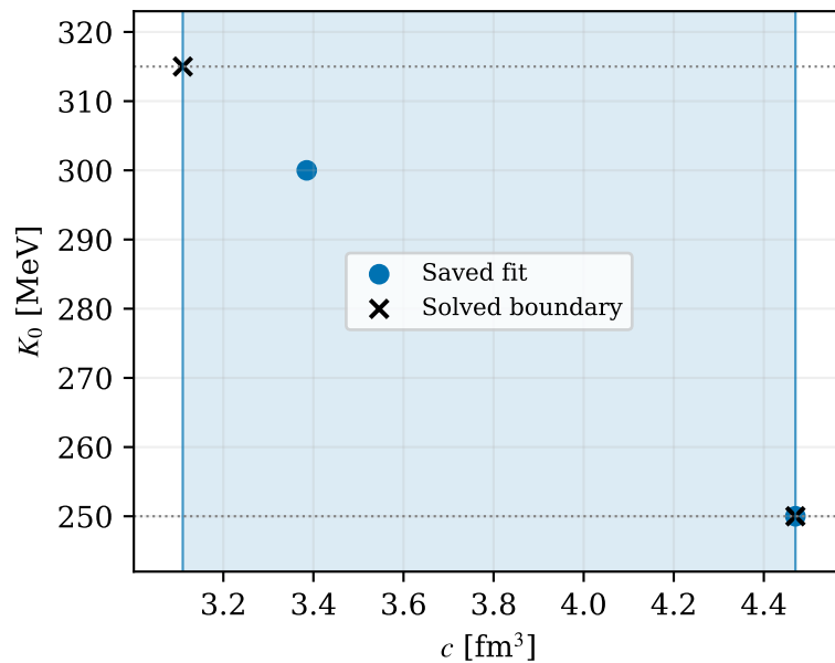
Clausius-CS
