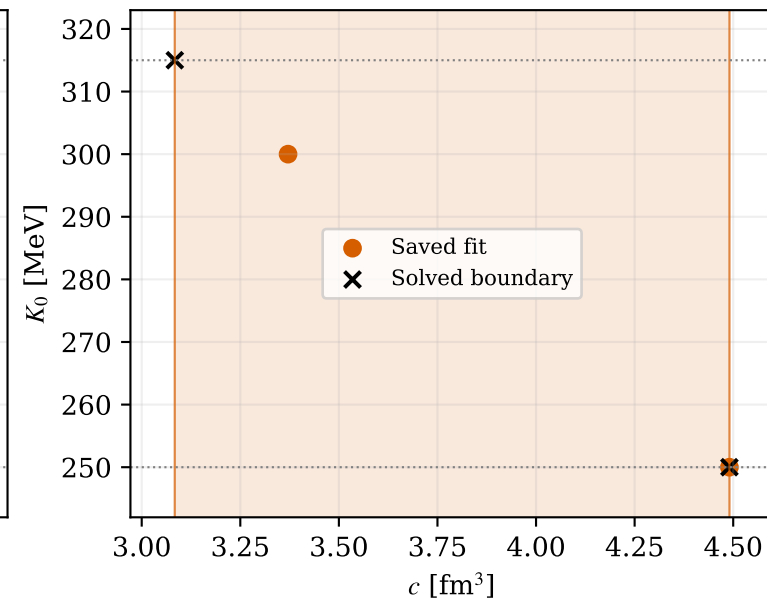
Clausius-TVM
