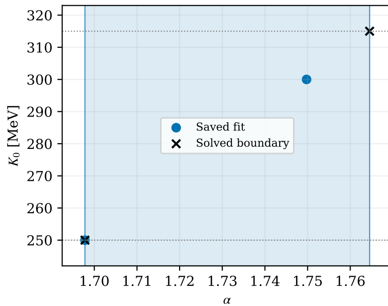
Clausius-CS
