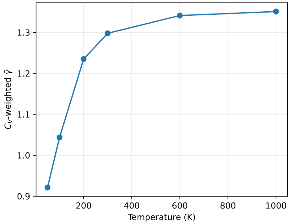
Thermodynamic Gruneisen parameter
