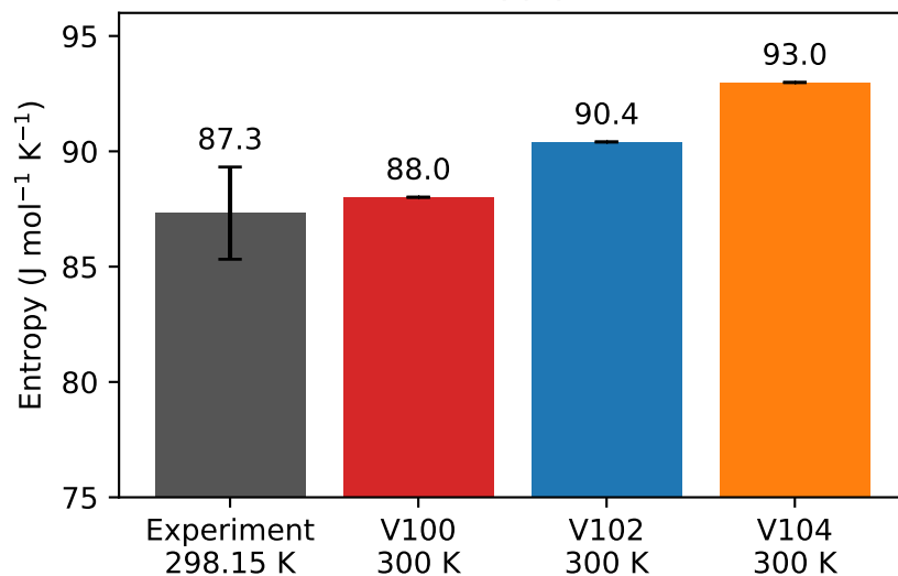
Molar entropy per Fe 2 O 3
