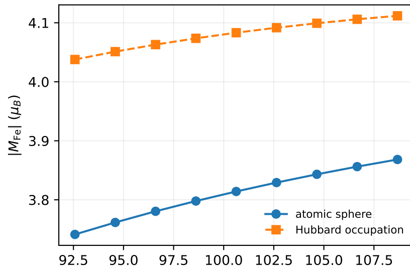
Fe local moment
