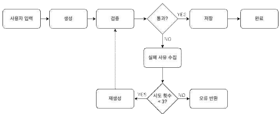
[그림 1. 검증·재생성 파이프라인 흐름]
