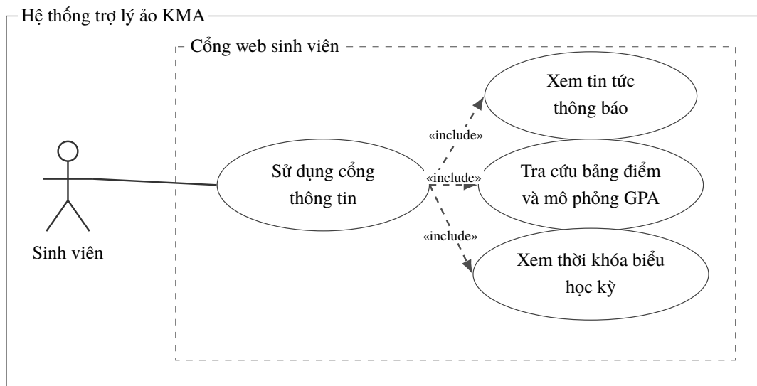
Hình 3.11 Use case sử dụng cổng thông tin
