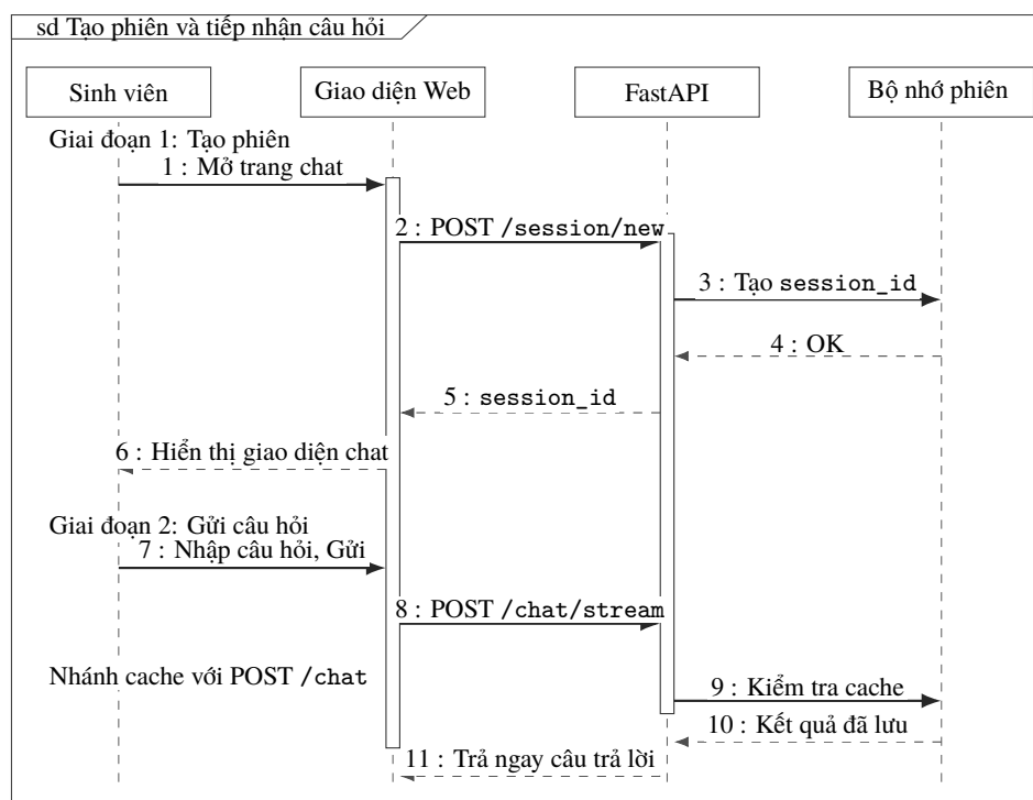
Hình 3.13 Biểu đồ tuần tự giai đoạn tạo phiên và tiếp nhận câu hỏi
