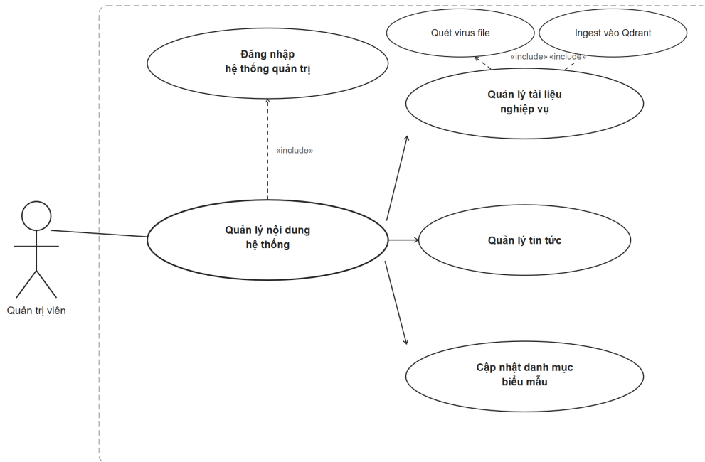
Hình 3.12 Use case quản lý nội dung hệ thống
