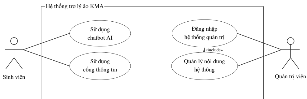
Hình 3.1 Biểu đồ use case tổng quát của hệ thống
