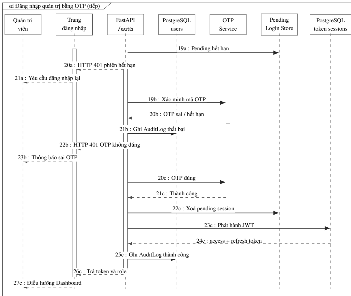
Hình 3.20 Biểu đồ tuần tự luồng xác thực OTP và phát hành JWT
