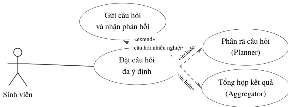
Hình 3.7 Use case đặt câu hỏi đa ý định
