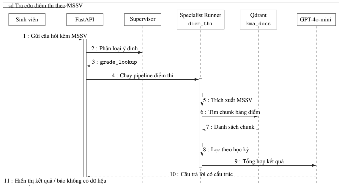
Hình 3.16 Biểu đồ tuần tự luồng tra cứu điểm thi theo MSSV
