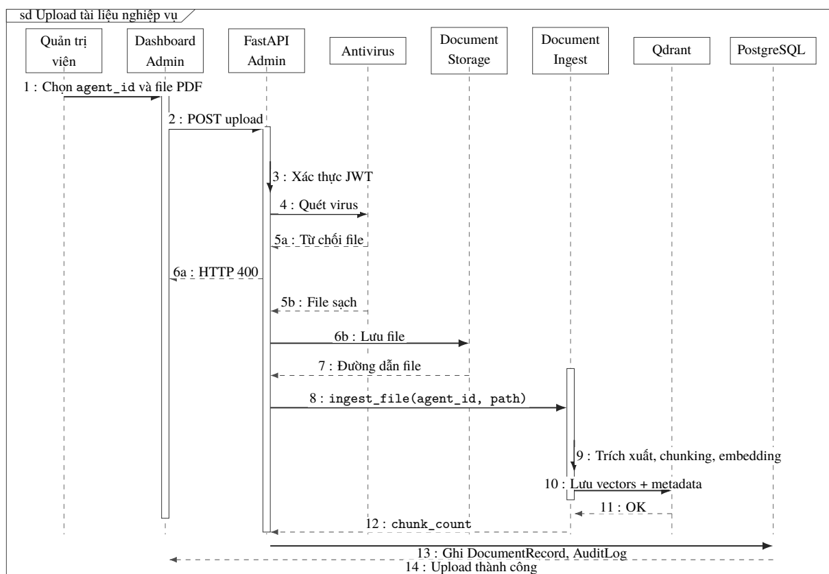
Hình 3.18 Biểu đồ tuần tự luồng upload tài liệu nghiệp vụ
