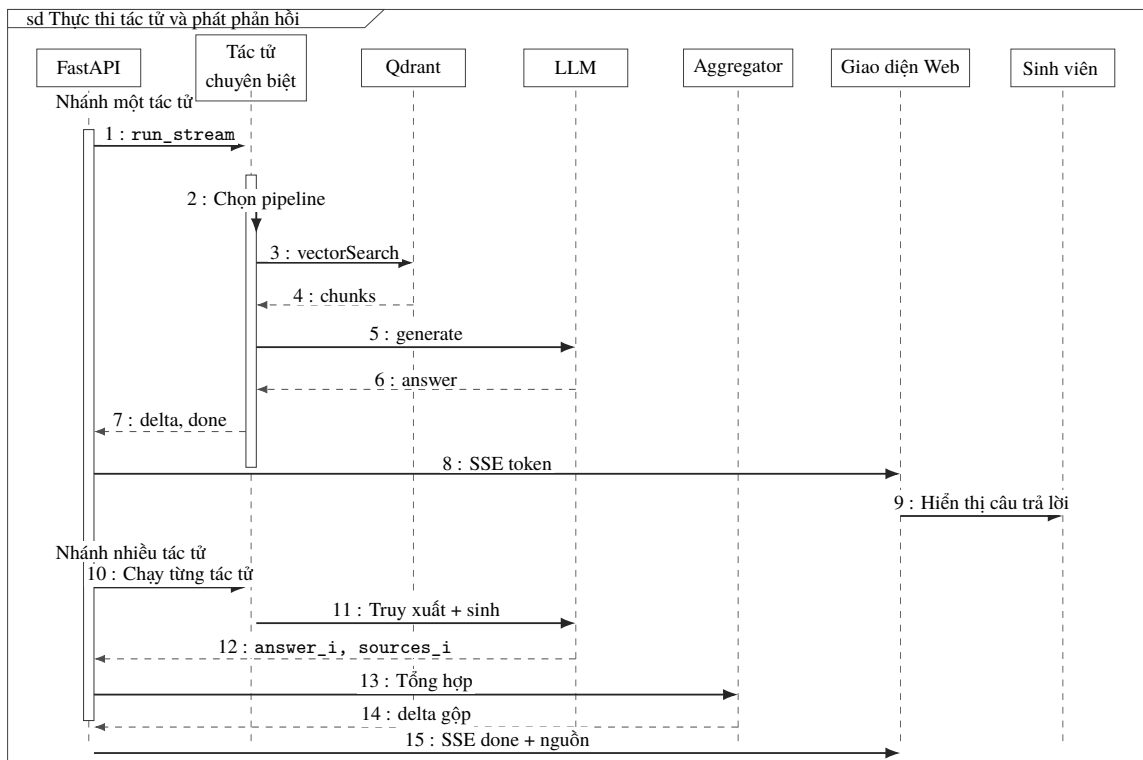
Hình 3.15 Biểu đồ tuần tự giai đoạn thực thi tác tử, truy xuất tri thức và phát phản hồi
