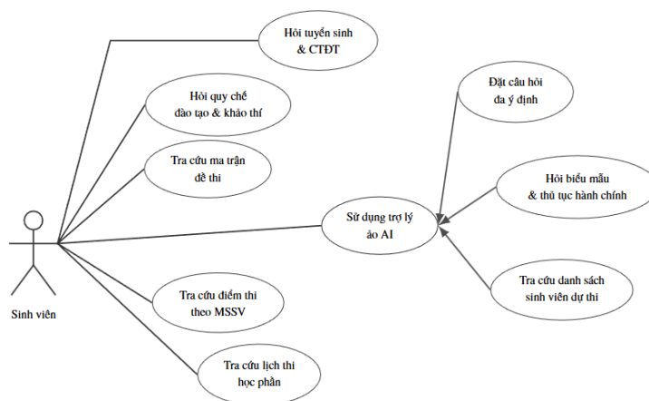
Hình 3.2 Use case gửi câu hỏi và nhận phản hồi từ chatbot
