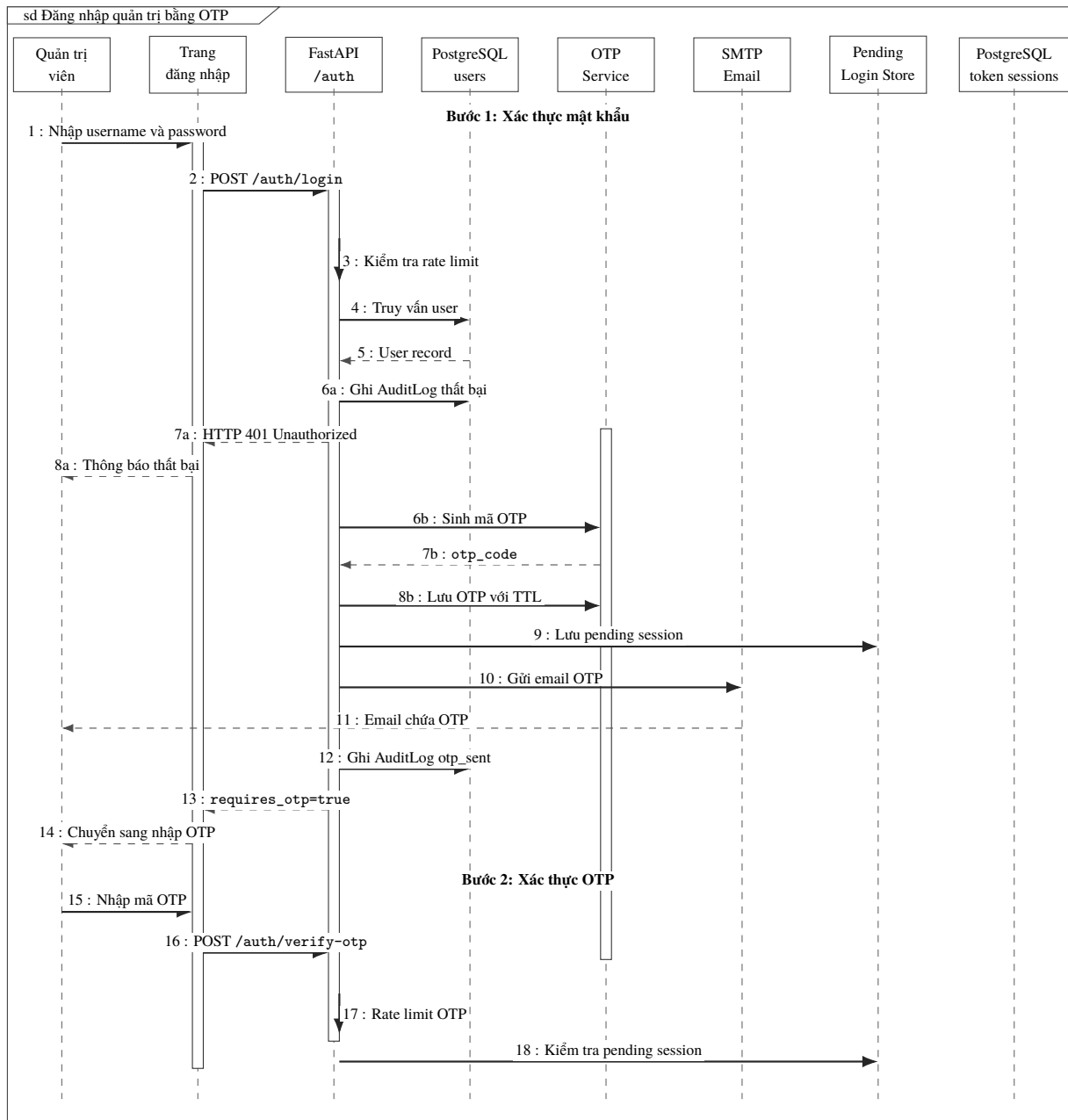
Hình 3.19 Biểu đồ tuần tự luồng đăng nhập hệ thống quản trị bằng OTP
