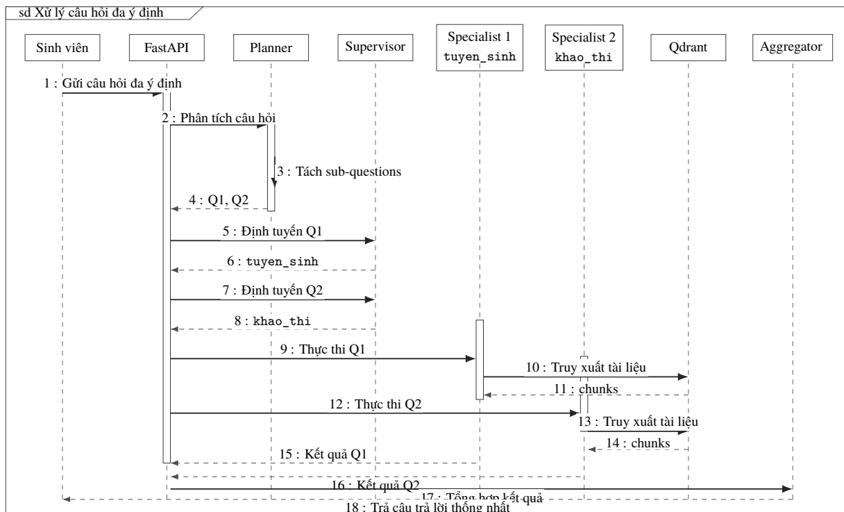
Hình 3.17 Biểu đồ tuần tự luồng xử lý câu hỏi đa ý định
