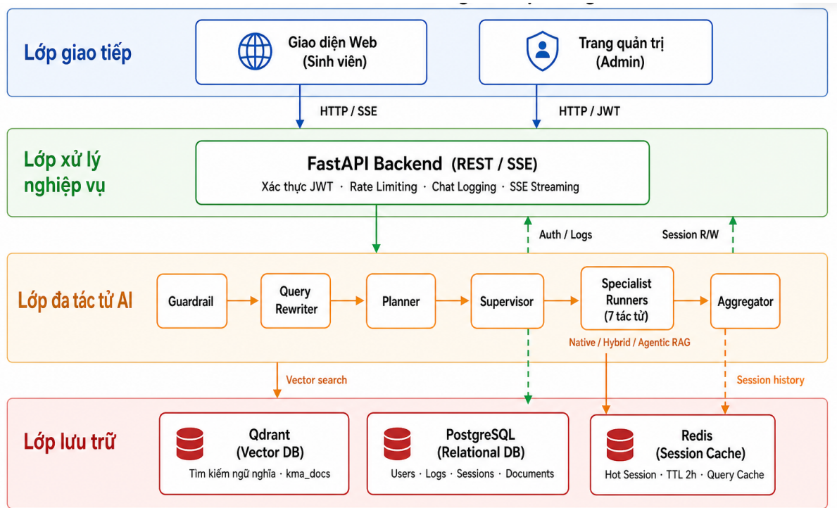
Hình 3.21 Sơ đồ kiến trúc tổng thể hệ thống
