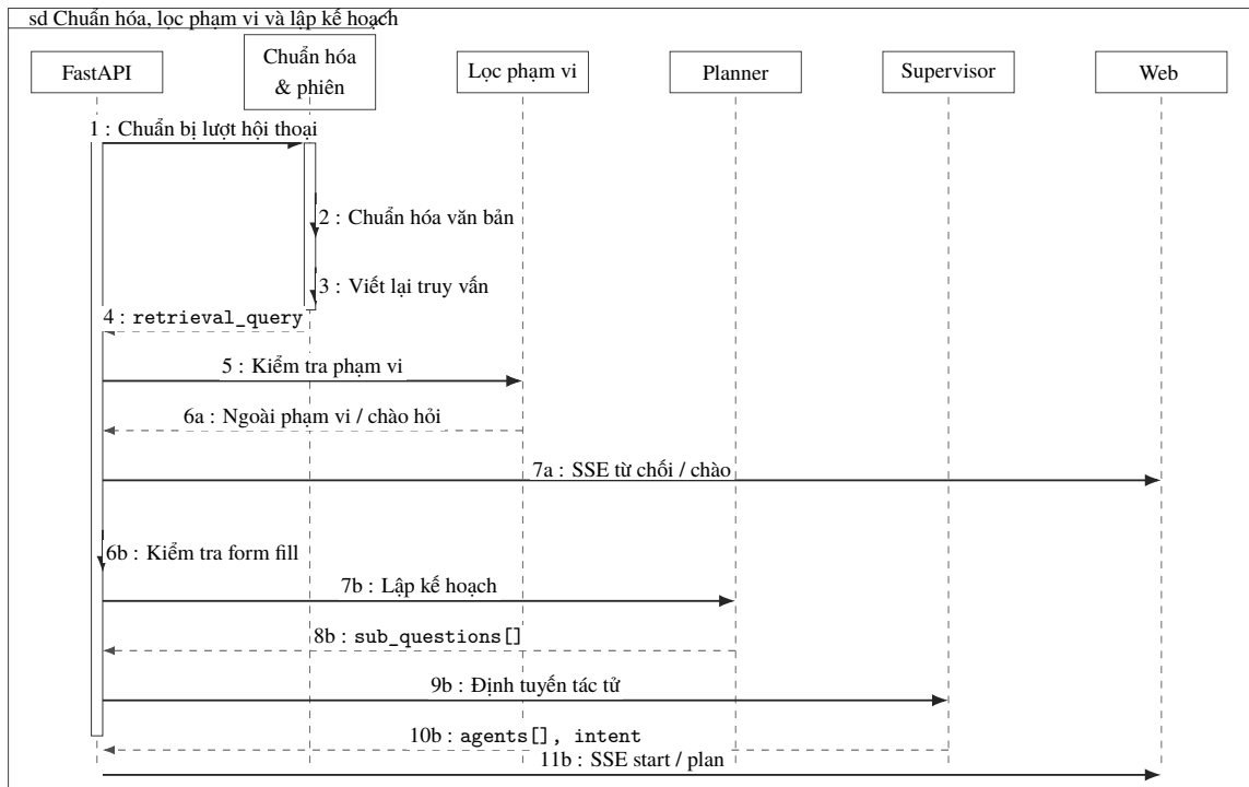
Hình 3.14 Biểu đồ tuần tự giai đoạn chuẩn hóa, lọc phạm vi và lập kế hoạch định tuyến
