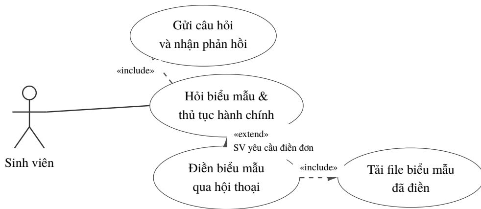
Hình 3.6 Use case hỏi biểu mẫu và thủ tục hành chính
