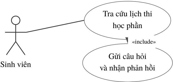
Hình 3.4 Use case tra cứu lịch thi học phần
