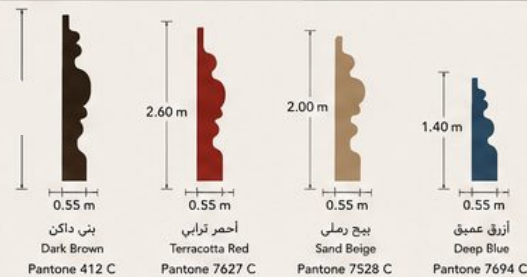
ألوان وقياسات الألواح الجدارية (الديكور الرئيسي) Wall Panel Pattern - Colors & Dimensions
