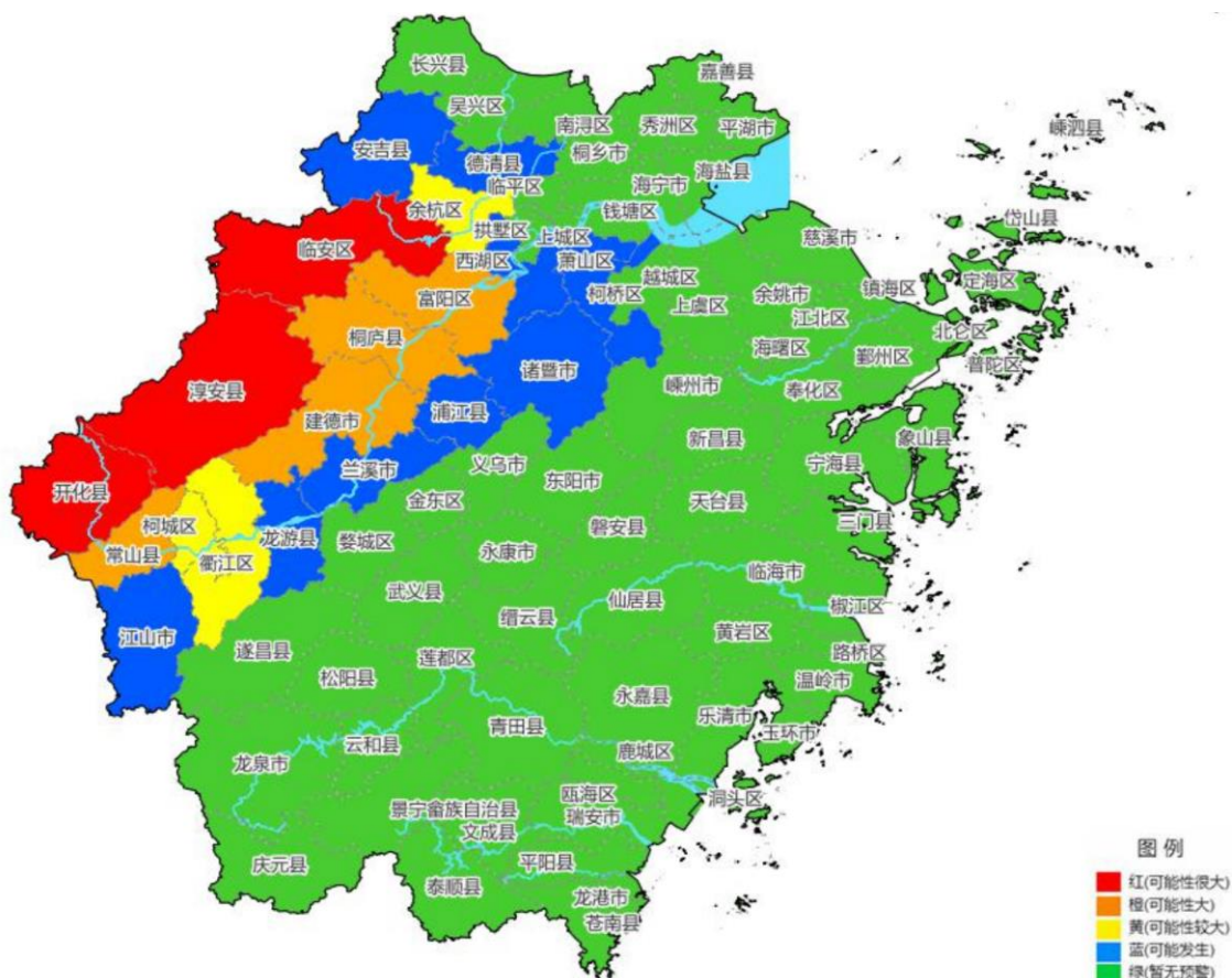
图 1 2024 年第 45 期 24 小时山洪预报预警图
