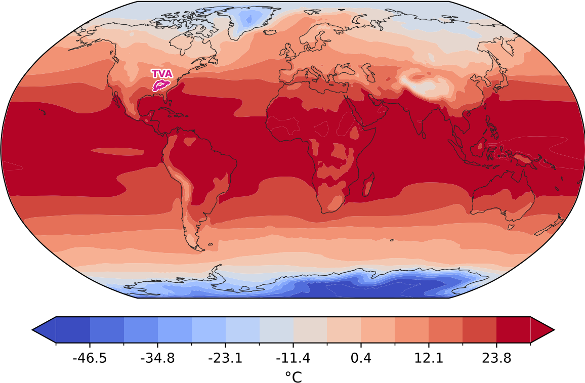
(b) E3SM v3
