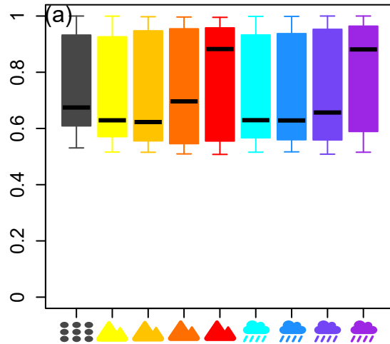
Precision
