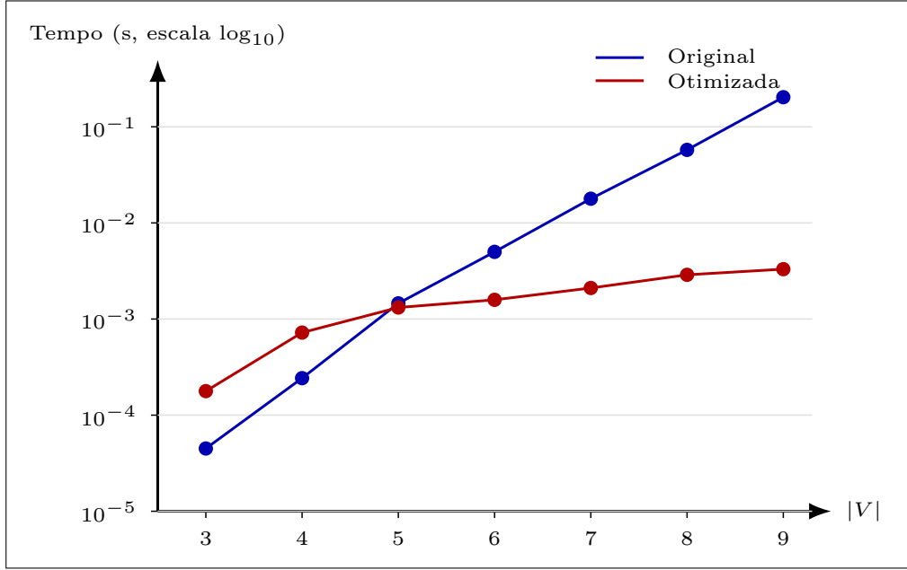
Figura 4: Tempos observados em grafos completos K_n
