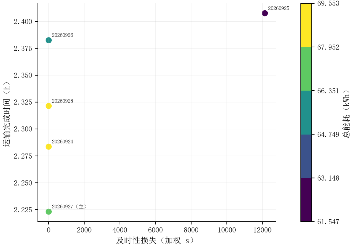
多种子解的及时性—完成时间—能耗权衡
