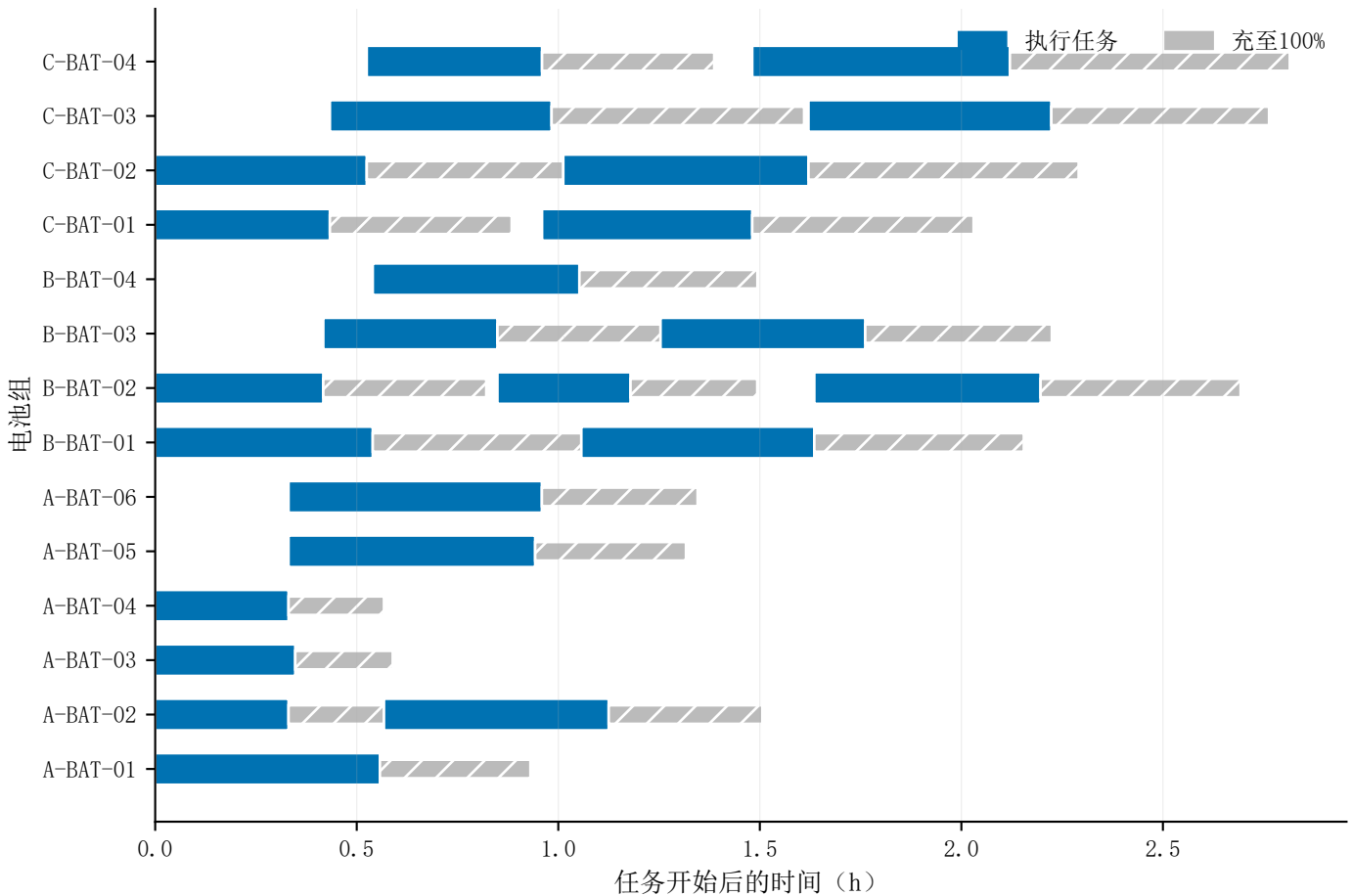
S2 主方案电池任务占用与两阶段充电
