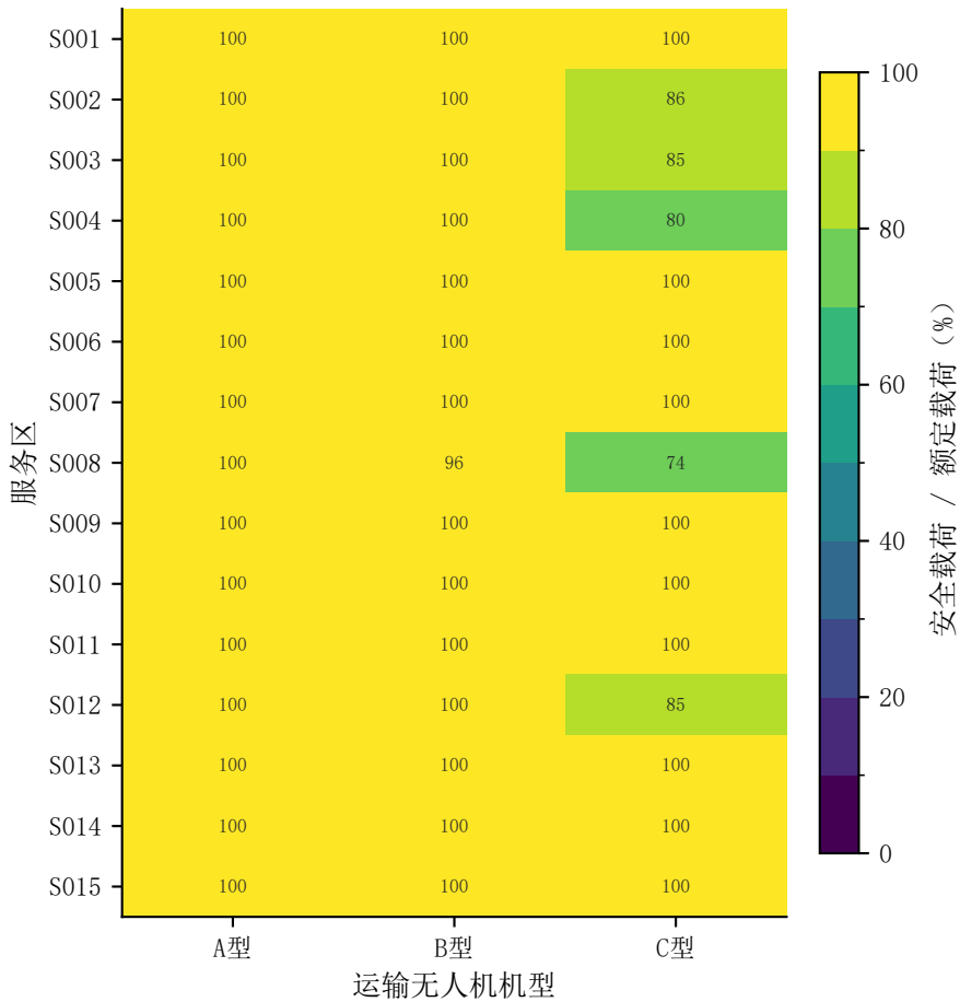
20%返航余量下最大安全载荷占额定载荷比例
