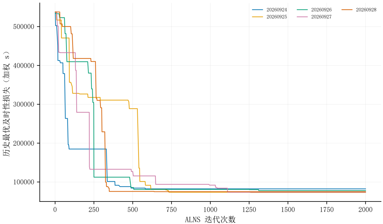
5 个固定随机种子的 ALNS 收敛轨迹
