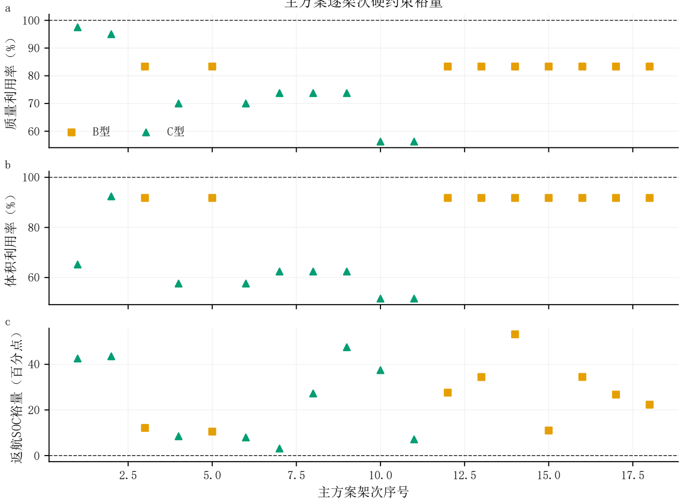
主方案逐架次硬约束裕量
