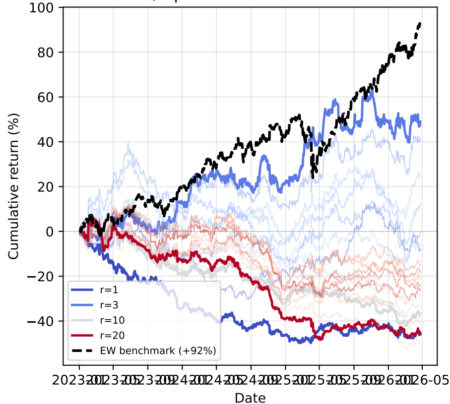
L/S portfolio actual returns
