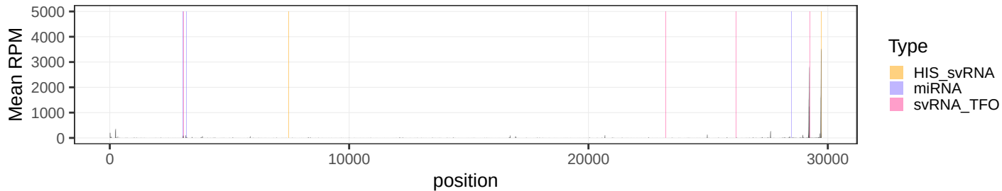
SARS-CoV-1
