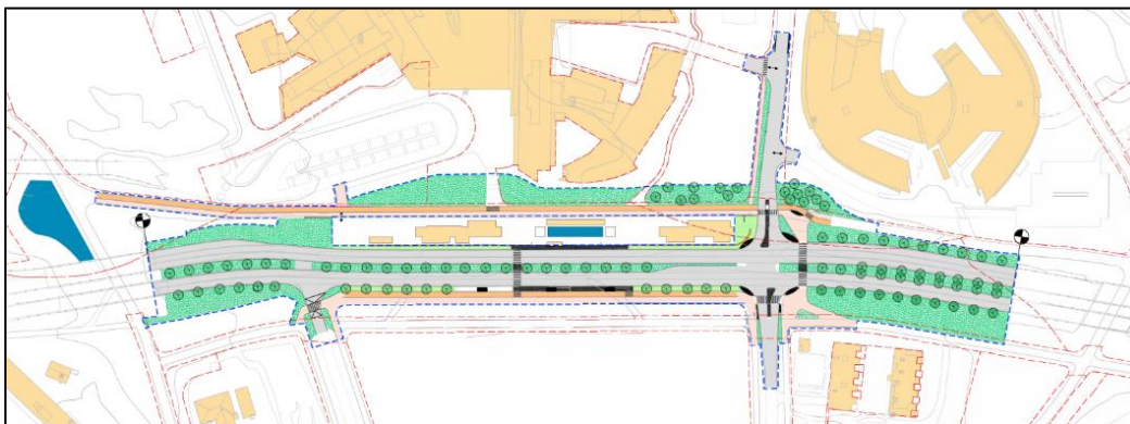
Figur 4-2 Tegning som viser strekningen av Snarøyveien som inngår i detaljreguleringsplanen (kilde: FOB/PGF).
