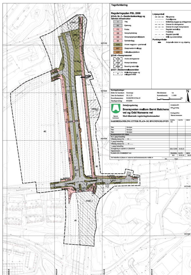
Figur 4-3 Foreslått plankart med planområde etter reduksjon av prosjektområdet (kilde: FOB/PGF).
