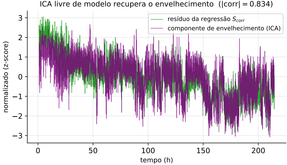
Figura 6: O componente de envelhecimento recuperado pelo ICA (roxo) sobreposto ao resíduo baseado em regressão S_{corr} (verde), ambos padronizados ( z -score). O ICA livre de modelo, dado apenas (S, T, V) , acompanha o sinal de envelhecimento da regressão em |corr| = 0.834 .
