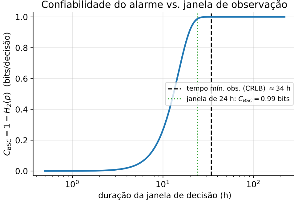
Figura 3: Capacidade do canal de alarme de envelhecimento C_{BSC} = 1 - H_2(p) em função do comprimento da janela de decisão. A confiabilidade sobe de \approx 0 (por hora, enterrada no ruído) para \approx 1 bit, com a transição coincidindo com o tempo mínimo de observação de Cramér–Rao ( \approx 34 h, tracejado) — as três figuras de mérito são mutuamente consistentes.
