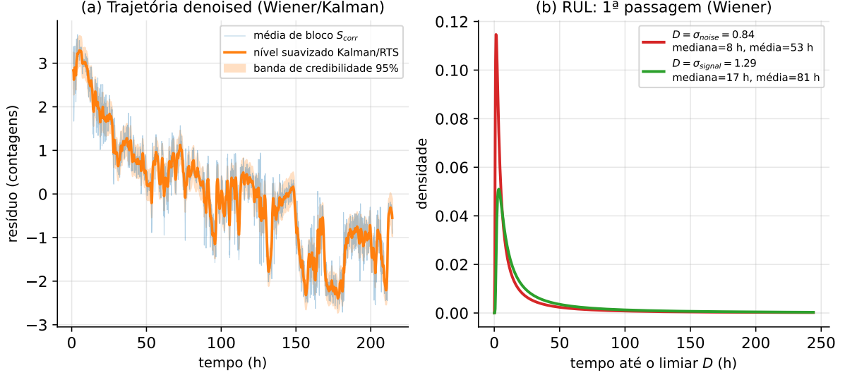
Figura 4: (a) Média de bloco de S_{\text{corr}} (claro) e a trajetória de envelhecimento suavizada por Kalman/RTS \hat{X}(t) com uma banda de credibilidade de 95%. (b) A distribuição de RUL Gaussiana-inversa (eq. (13)) em dois limiares ancorados no Tier 1: um incremento do piso de ruído ( D = \sigma_{\text{noise}} ) e uma excursão em escala de sinal já observada ( D = \sigma_{\text{signal}} ).
