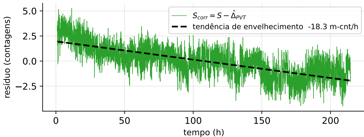
(b) Após correção PVT: envelhecimento exposto (corr c/ tempo -0.35 \rightarrow -0.73 )
