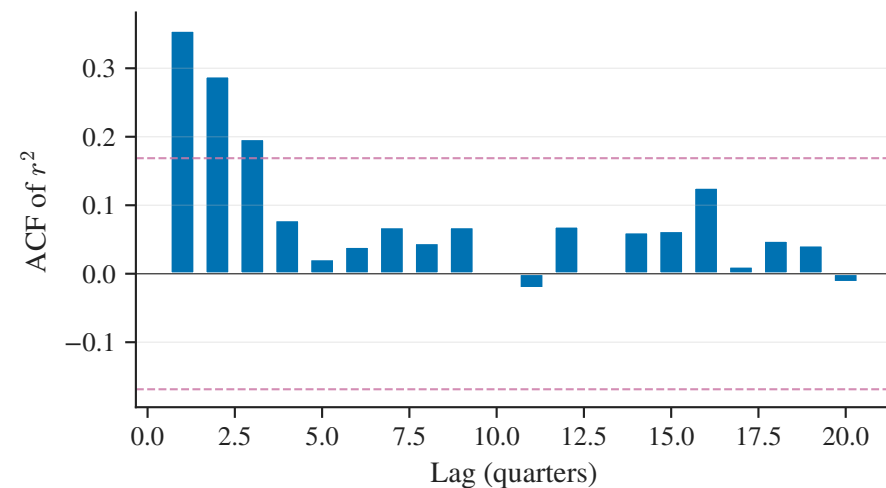
(d) Volatility clustering check (Paris)
