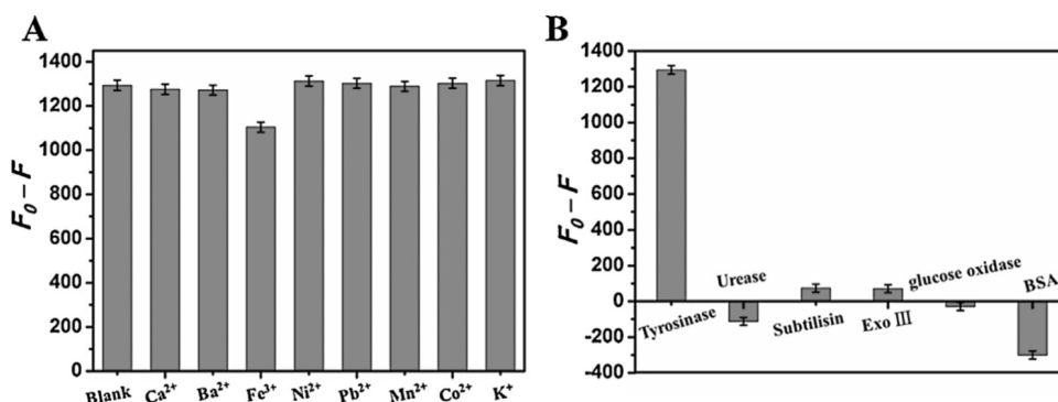
Рисунок 10: Графики зависимости снижения интенсивности флуоресценции ( F_0 - F ) для золотых нанокластеров, стабилизированных тирозином, в присутствии: (A) ионов биологически значимых металлов (добавленных в концентрации 250 мкМ) при присутствии в растворе тирозиназы (50 ед/мл); (B) тирозиназы, уреазы, субтилизины, экзонуклеазы III, глюкозооксидазы (по 50 ед/мл) и бычьего сывороточного альбумина (1 мг/мл) соответственно [1].
