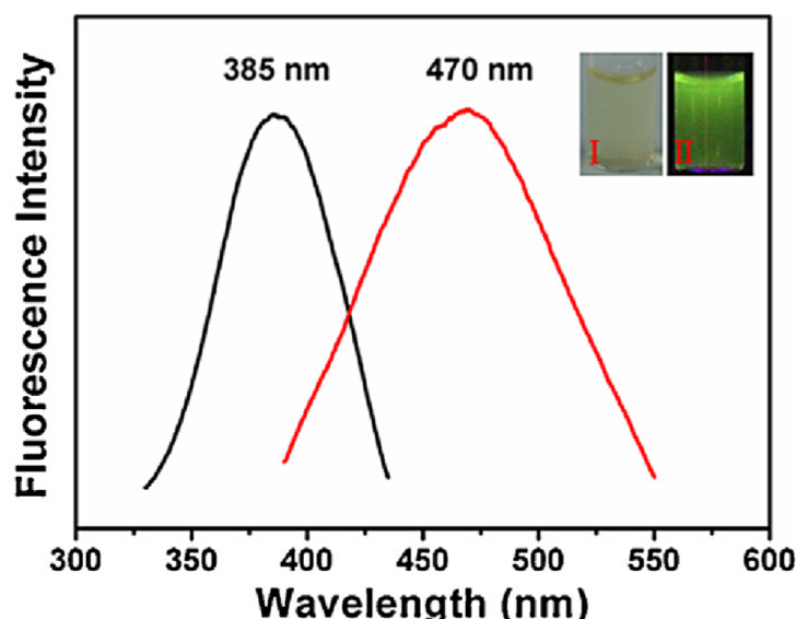
Рисунок 9: Спектры возбуждения (чёрная линия) и эмиссии флуоресценции (красная линия) тирозин-стабилизированного золотого нанокластера. На вставке: фотографии кластера при дневном освещении (I) и в ультрафиолетовом свете (II). [1]
