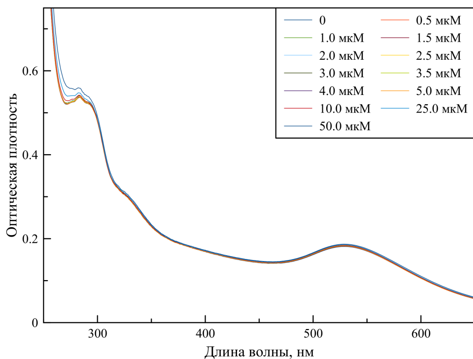
Рисунок 29: Спектры поглощения перерастворённого тирозин-стабилизированного золотого нанокластера после лиофилизации в присутствии ионов меди.
