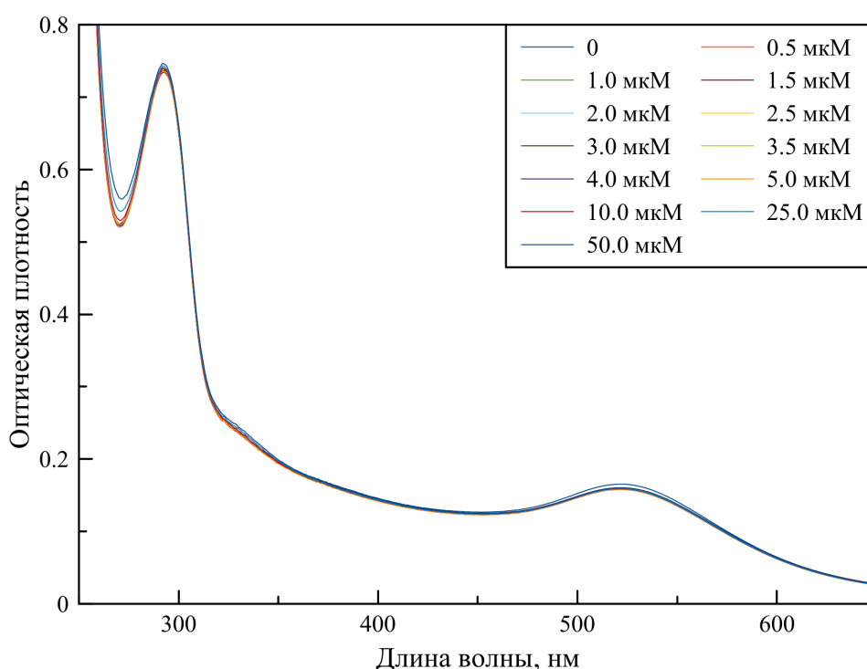
Рисунок 24: Спектры поглощения золотого нанокластера, стабилизированного тирозином, в присутствии ионов меди. Стрелка указывает направление увеличения концентрации аналита
