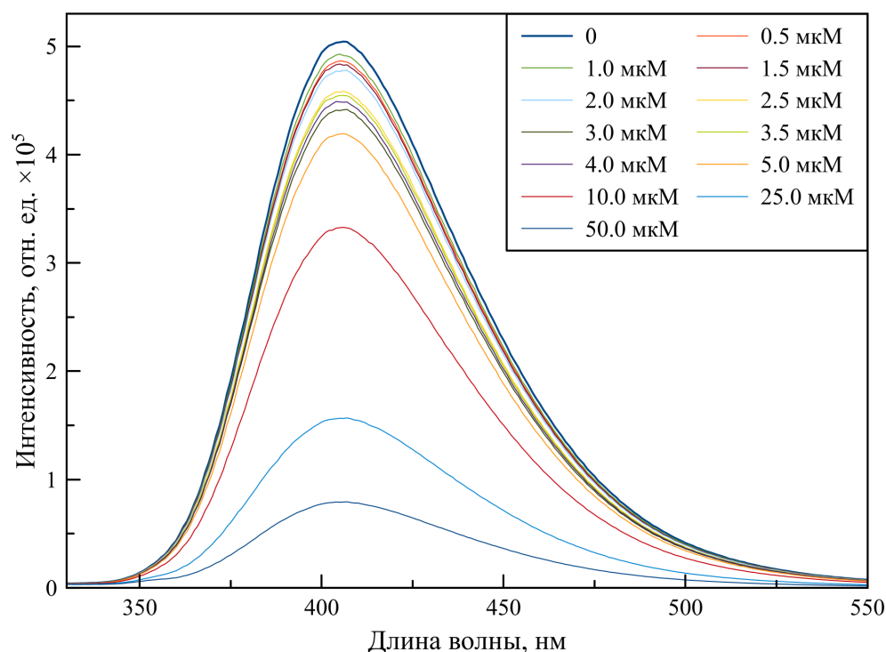
Рисунок 30: Скорректированные спектры испускания перерастворённого тирозин-стабилизированного золотого нанокластера после лиофилизации в присутствии ионов меди ( \lambda_{\text{возб}} = 315 нм)
