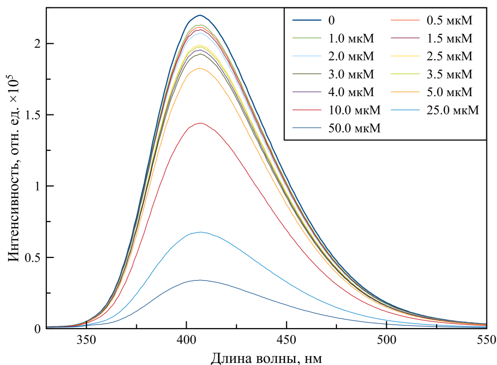
Рисунок 29: Спектры испускания перерастворённого AuNCs@Tyr после лиофилизации в присутствии ионов меди ( \lambda_{\text{возб}} = 315 нм). Стрелка указывает направление увеличения концентрации аналита
