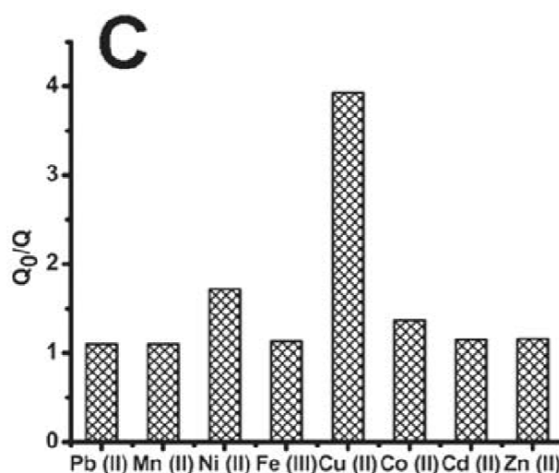
Рисунок 13: Относительная интенсивность люминесценции БСА-стабилизированного золотого нанокластера в присутствии ионов тяжелых металлов [24].
