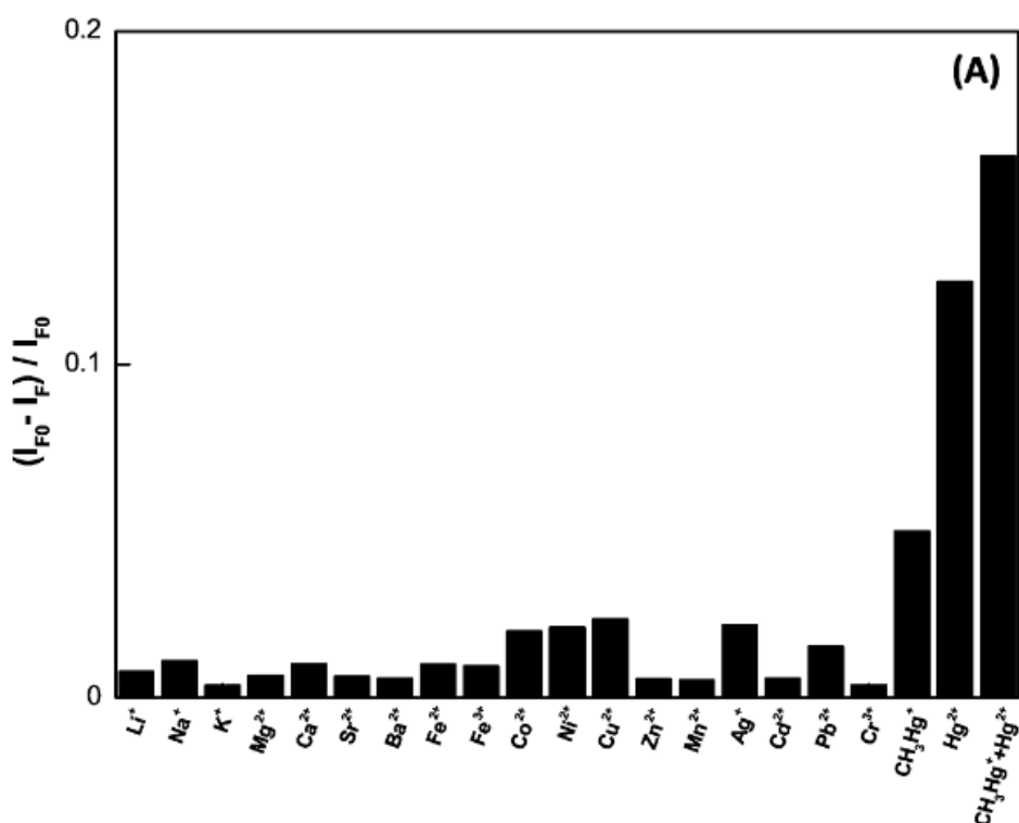
Рисунок 11: Относительная интенсивность люминесценции золотого нанокластера, стабилизированного лизоцимом-VI в присутствии ионов металлов в концентрации 50 мкмоль [23].
