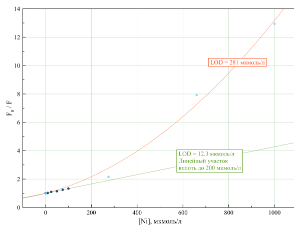
Рис. 12: График Штерна-Фольмера для никеля
