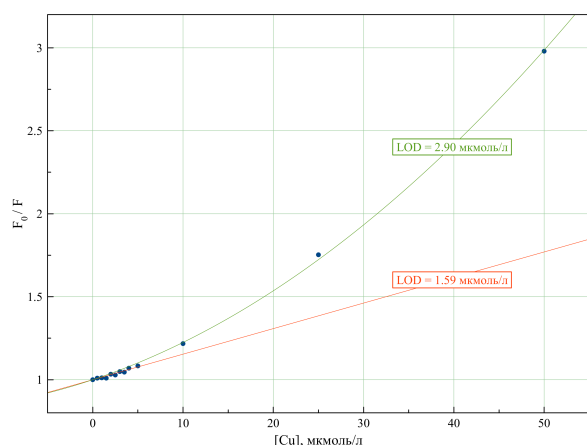
Рис. 11: График Штерна-Фольмера для меди
