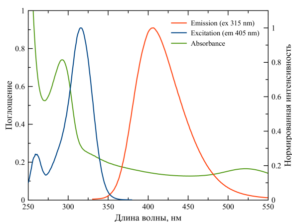
Рис. 8: Спектры поглощения, возбуждения и испускания золотых нанокластеров
