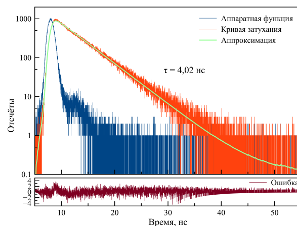
Рис. 9: Кривая затухания люминесценции золотого нанокластера
