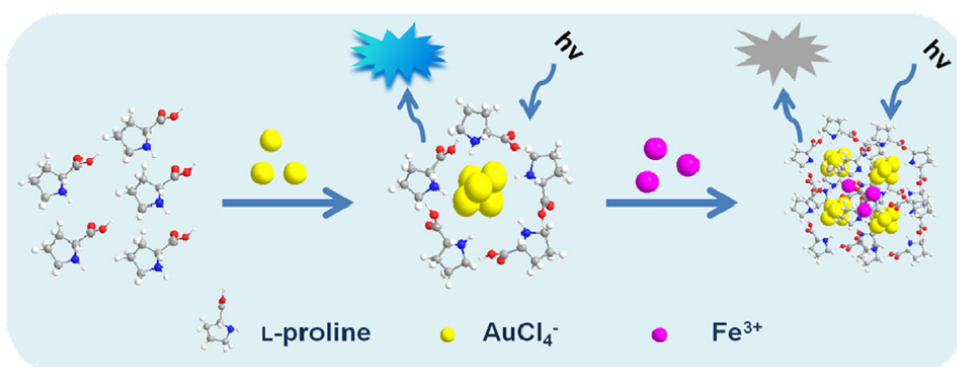
Рис. 6: Схема синтеза золотых наночастиц на L-пролине для последующей детекции ионов железа [9]
