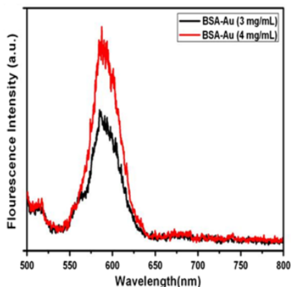
Рис. 4: Спектры флюоресценции золотых нанокмплексов, стабилизированных БСА с различной концентрацией на длине возбуждения 470 нм [3]
