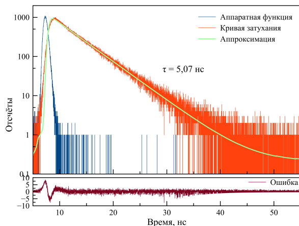
Рис. 13: Время жизни люминесценции в присутствии меди
