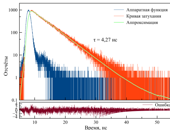
Рис. 14: Время жизни люминесценции в присутствии никеля
