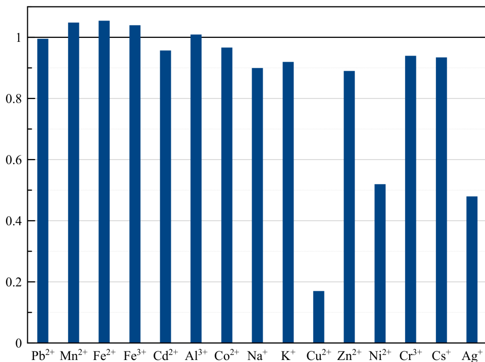
Рис. 10: Изменение люминесценции кластера в присутствии ионов металлов в концентрации 100 ммоль/л
