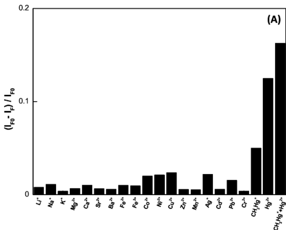
Рис. 9: Относительная интенсивность люминесценции золотого нанокластера, стабилизированного лизоцимом-VI в присутствии ионов металлов в концентрации 50 мкмоль [13]
