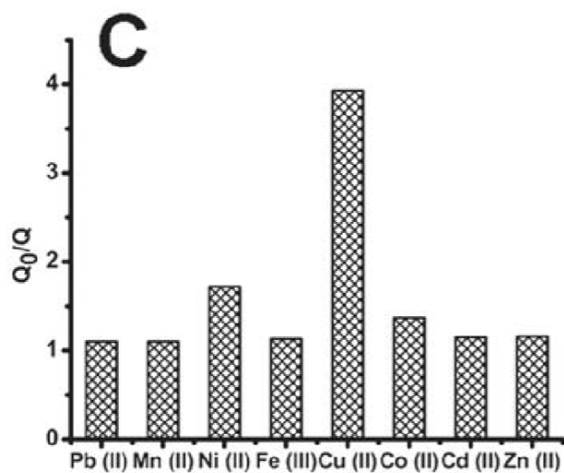
Рис. 11: Относительная интенсивность люминесценции БСА-стабилизированного золотого нанокластера в присутствии ионов тяжелых металлов [9]
