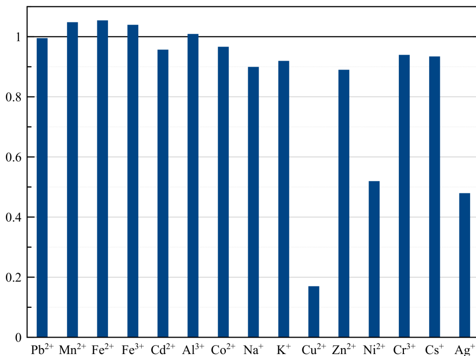
Рисунок 17: Изменение люминесценции кластера в присутствии ионов металлов в концентрации 100 мкмоль/л
