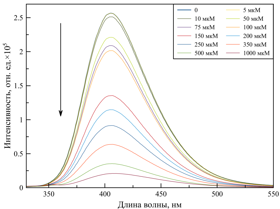
Рисунок 19: Спектры испускания золотого нанокластера, стабилизированного тирозином в присутствии ионов никеля, снятые при длине волны возбуждения равной 315 нм. Стрелка указывает в направлении увеличения концентрации аналита
