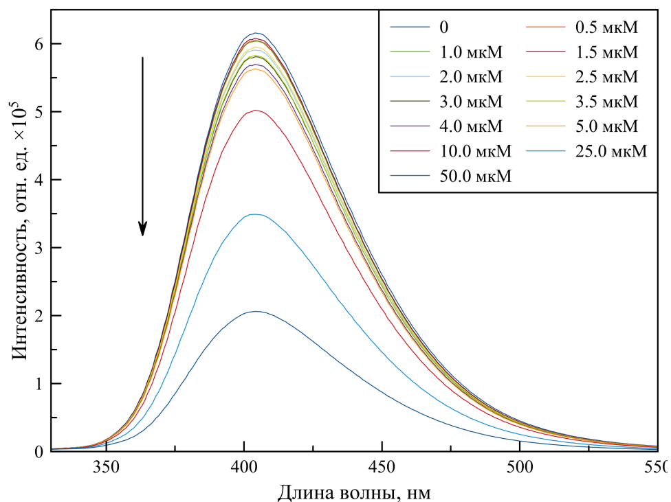
Рисунок 25: Скорректированные спектры испускания золотого нанокластера, стабилизированного тирозином, в присутствии ионов меди, снятые при длине волны возбуждения, равной 315 нм. Стрелка указывает направление увеличения концентрации аналита
