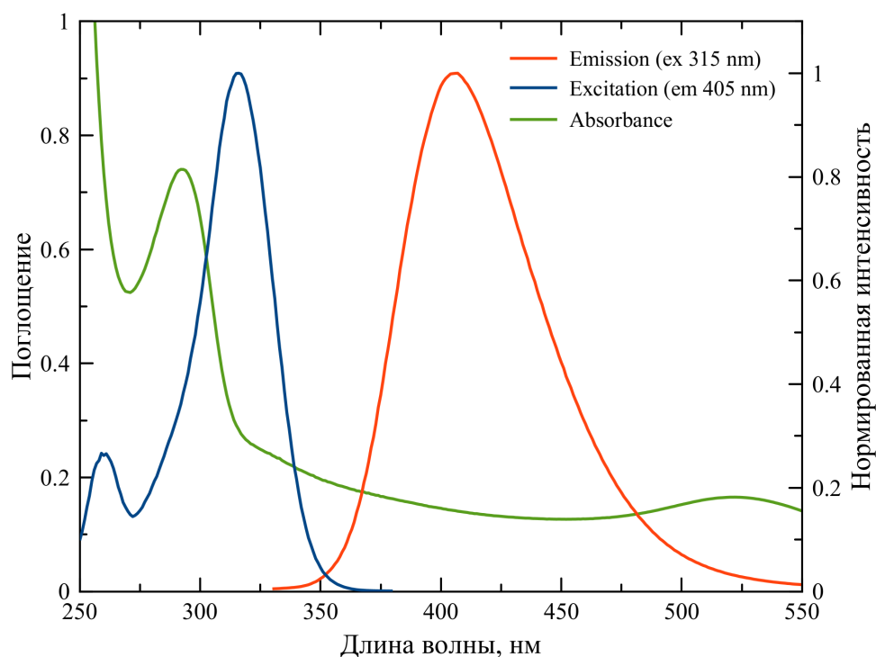
Рисунок 15: Спектры поглощения, возбуждения и испускания золотых нанокластеров
