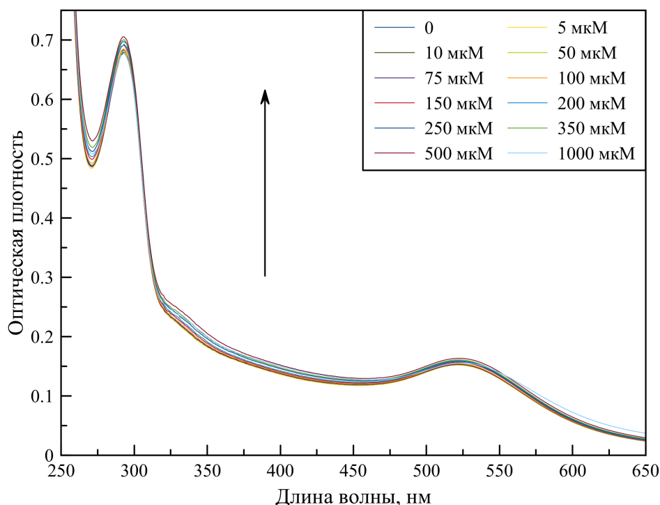
Рисунок 18: Спектры поглощения золотого нанокластера, стабилизированного тирозином в присутствии ионов никеля. Стрелка указывает в направлении увеличения концентрации аналита
