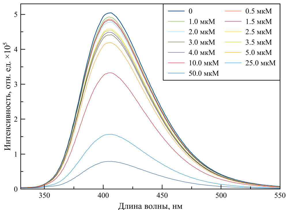
Рисунок 29: Скорректированные спектры испускания перерастворённого тирозин-стабилизированного золотого нанокластера после лиофилизации в присутствии ионов меди ( \lambda_{\text{возб}} = 315 \text{ нм} )
