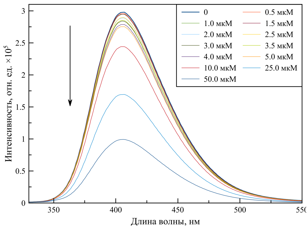
Рисунок 24: Спектры испускания золотого нанокластера, стабилизированного тирозином, в присутствии ионов меди, снятые при длине волны возбуждения, равной 315 нм. Стрелка указывает направление увеличения концентрации аналита
