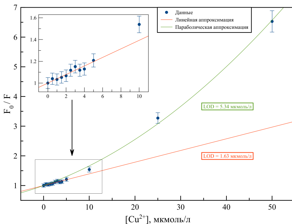
Рисунок 30: График Штерна-Фольмера для перерастворённого после лиофилизации AuNCs@Tyr в присутствии ионов меди
