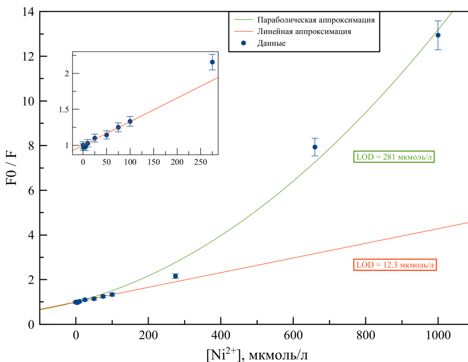
Рисунок 21: График Штерна-Фольмера для никеля
