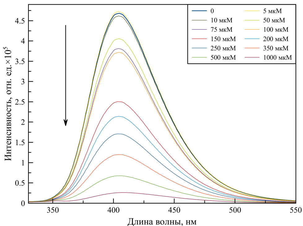
Рисунок 20: Корректированные спектры испускания золотого нанокластера, стабилизированного тирозином в присутствии ионов никеля, снятые при длине волны возбуждения равной 315 нм. Стрелка указывает в направлении увеличения концентрации аналита
