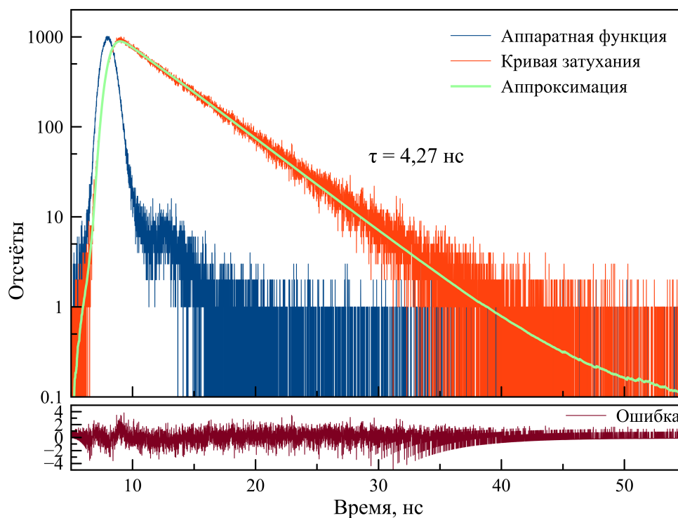
Рисунок 22: Кривая затухания люминесценции золотого нанокластера в присутствии ионов никеля в концентрации 100 мкмоль/л.
