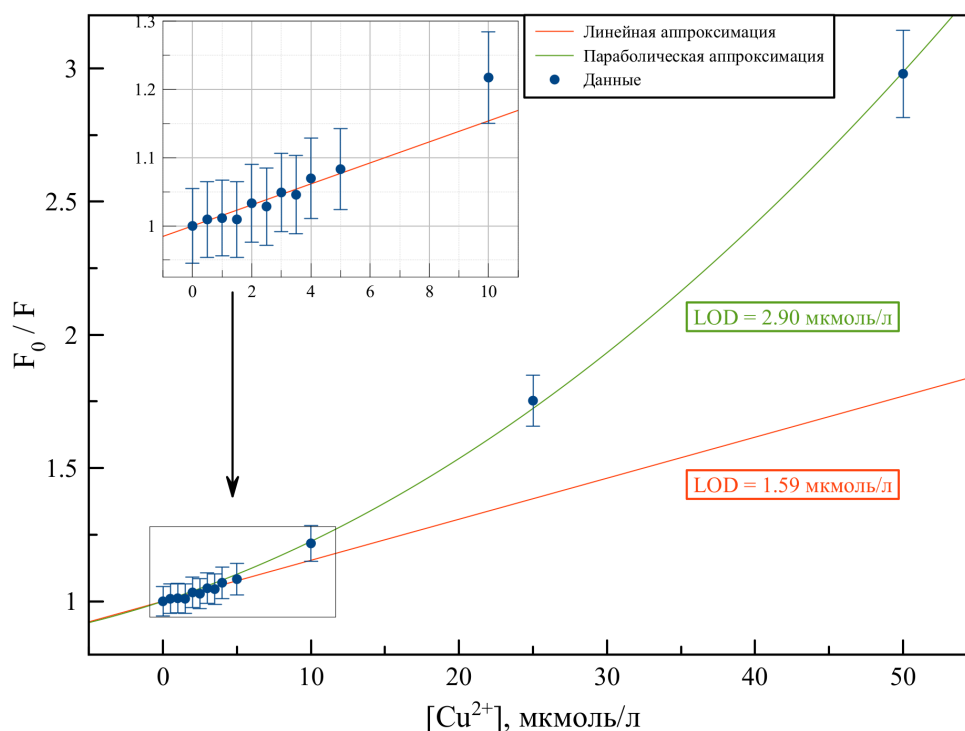
Рисунок 26: График Штерна-Фольмера для меди
