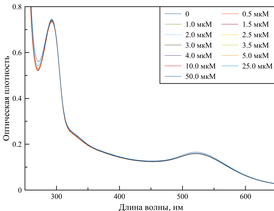
Рисунок 23: Спектры поглощения золотого нанокластера, стабилизированного тирозином, в присутствии ионов меди. Стрелка указывает направление увеличения концентрации аналита
