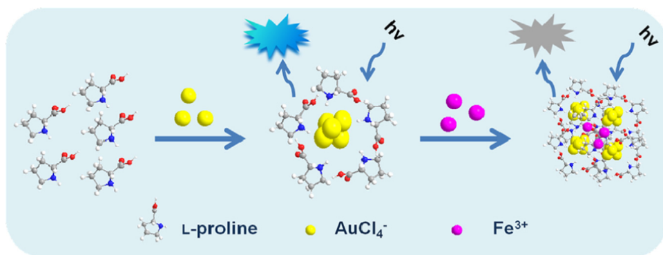
Рисунок 6: Схема синтеза золотых наночастиц на L-пролине для последующей детекции ионов железа [9]
