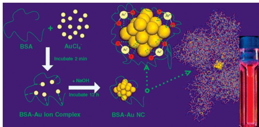
Рисунок 4: Схема образования золотых нанокластеров в растворе БСА [25]
