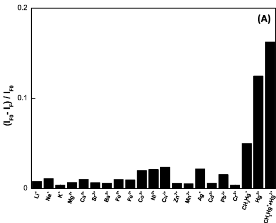
Рисунок 11: Относительная интенсивность люминесценции золотого нанокластера, стабилизированного лизоцимом-VI в присутствии ионов металлов в концентрации 50 мкмоль [14]
