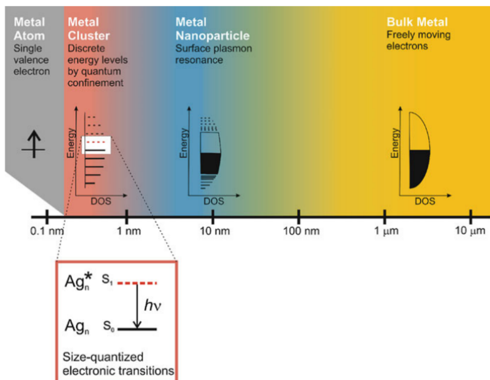
Рисунок 1: Сравнительная схема электронно-энергетических свойств металла в зависимости от его размера [6]
