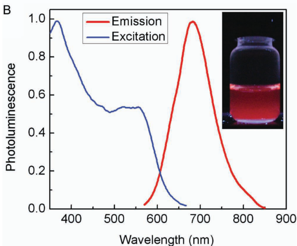
Рисунок 7: Спектры возбуждения и испускания золотого нанокластера, стабилизированного дигидролипоевой кислотой (DHLLA-AuNCs) [20]
