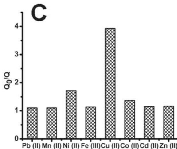
Рисунок 13: Относительная интенсивность люминесценции БСА-стабилизированного золотого нанокластера в присутствии ионов тяжелых металлов [8]
