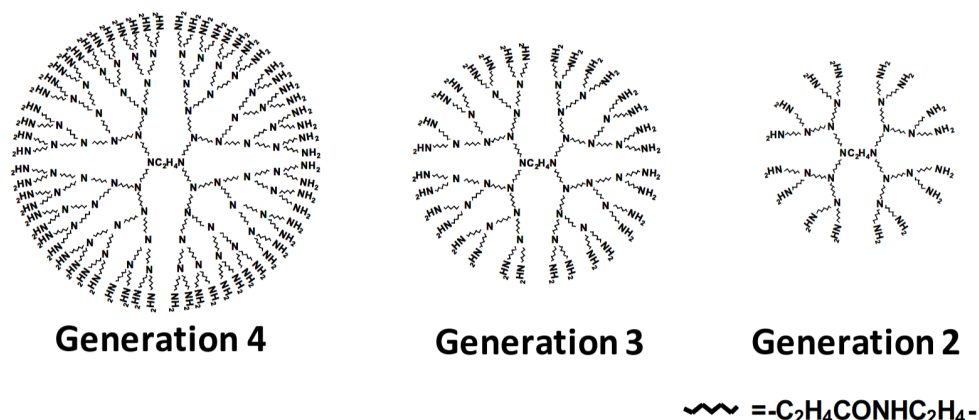
Рисунок 3: Химическая структура полиамидоаминов различных поколений [1]
