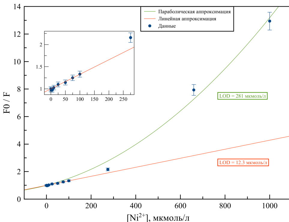
Рисунок 22: График Штерна-Фольмера для никеля
