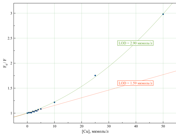
Рисунок 18: График Штерна-Фольмера для меди
