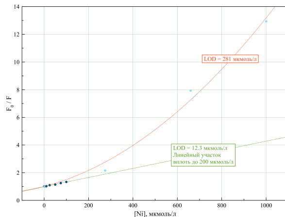
Рисунок 19: График Штерна-Фольмера для никеля
