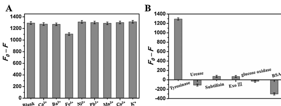
Рисунок 10: Графики зависимости снижения интенсивности флуоресценции ( F_0 - F ) для золотых наноклаusters, стабилизированных тирозином, в присутствии: (A) ионов биологически значимых металлов (добавленных в концентрации 250 мкМ) при присутствии в растворе тирозиназы (50 ед/мл); (B) тирозиназы, уреазы, субтилизина, экзонуклеазы III, глюкозооксидазы (по 50 ед/мл) и бычьего сывороточного альбумина (1 мг/мл) соответственно. [20]
