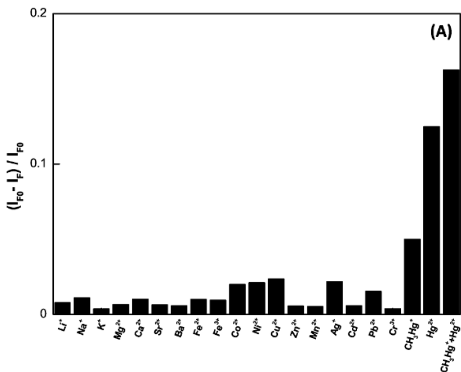
Рисунок 11: Относительная интенсивность люминесценции золотого нанокластера, стабилизированного лизоцимом-VI в присутствии ионов металлов в концентрации 50 мкмоль [15]
