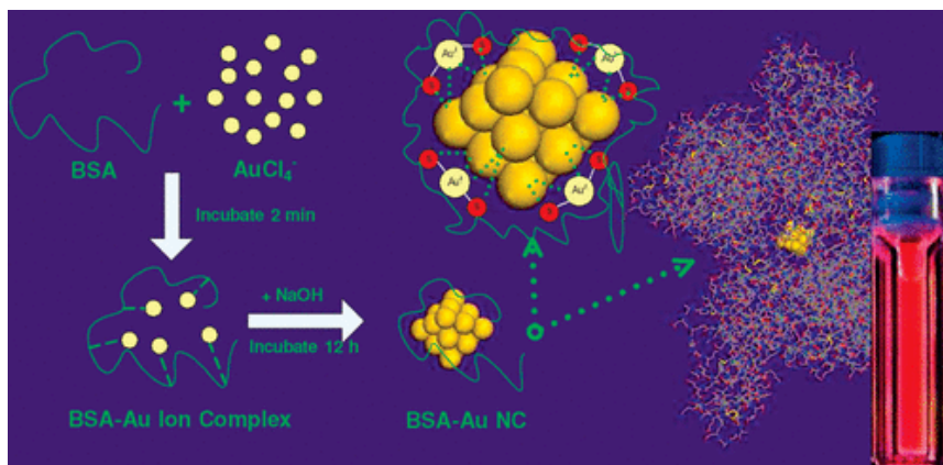
Рисунок 4: Схема образования золотых нанокластеров в растворе БСА [28]
