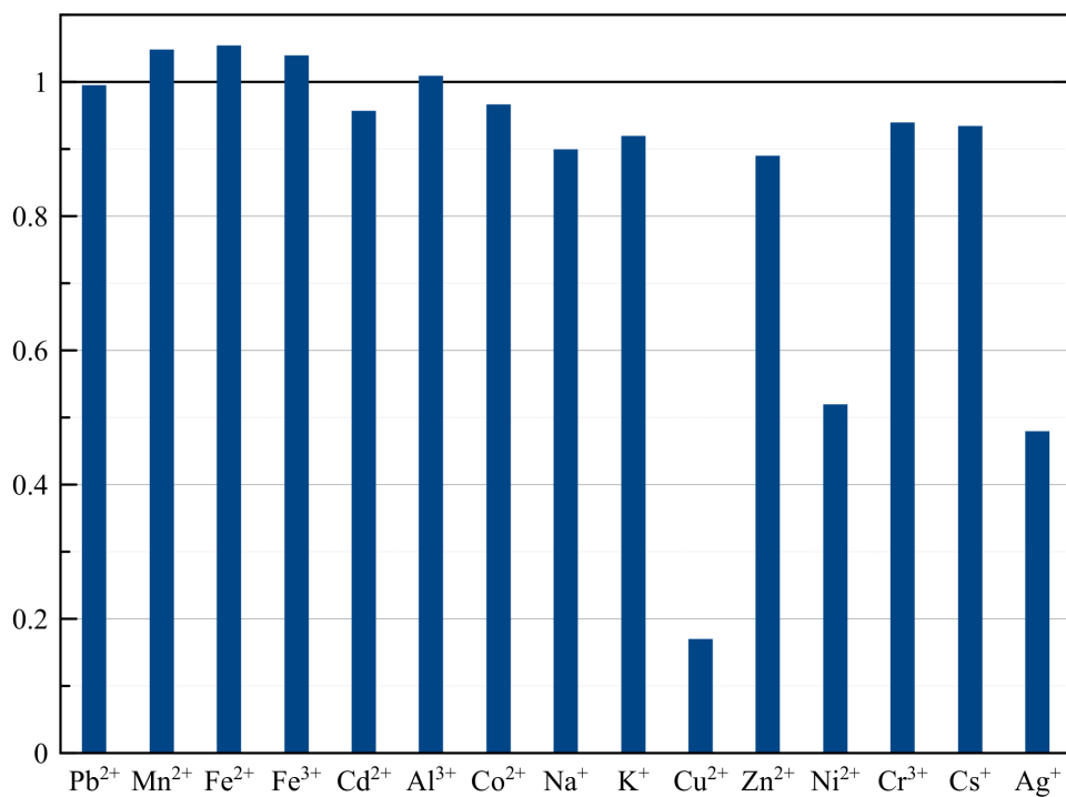
Рисунок 17: Изменение люминесценции кластера в присутствии ионов металлов в концентрации 100 ммоль/л
