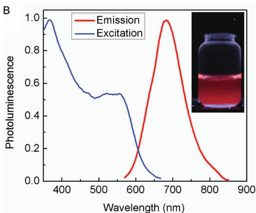
Рисунок 7: Спектры возбуждения и испускания золотого нанокластера, стабилизированного дигидролипоевой кислотой (DHLLA-AuNCs) [22]
