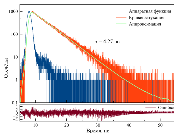
Рисунок 21: Время жизни люминесценции в присутствии никеля
