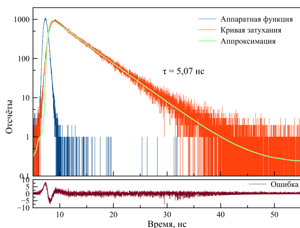
Рисунок 20: Время жизни люминесценции в присутствии меди
