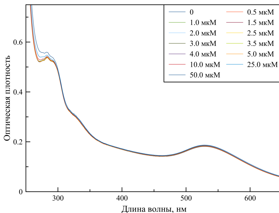
Рисунок 28: Спектры поглощения перерастворённого тирозин-стабилизированного золотого нанокластера после лиофилизации в присутствии ионов меди.
