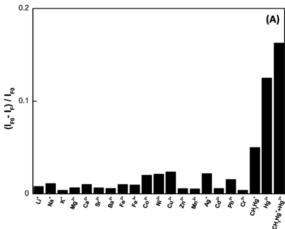
Рис. 9: Относительная интенсивность люминесценции золотого нанокластера, стабилизированного лизоцимом-VI в присутствии ионов металлов в концентрации 50 мкмоль [14]
