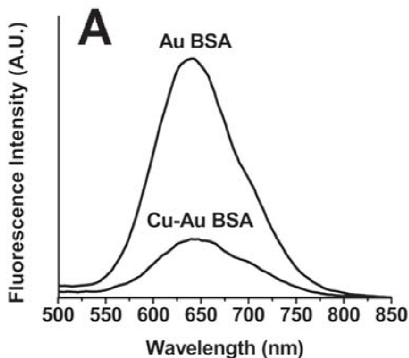
Рис. 10: Спектр исходной люминесценции БСА-стабилизированного золотого НК и после добавления тушителя (75 мкмоль Cu^{2+} ) с пиком в 645 нм при длине волны возбуждения 480 нм [9]
