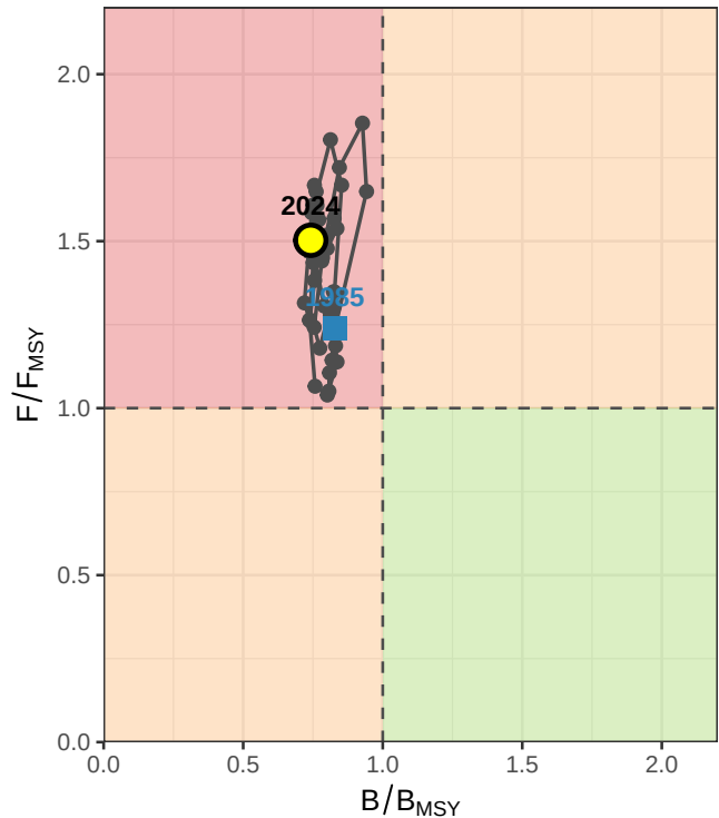
Kobe Plot: 1985 Lorenzen M
