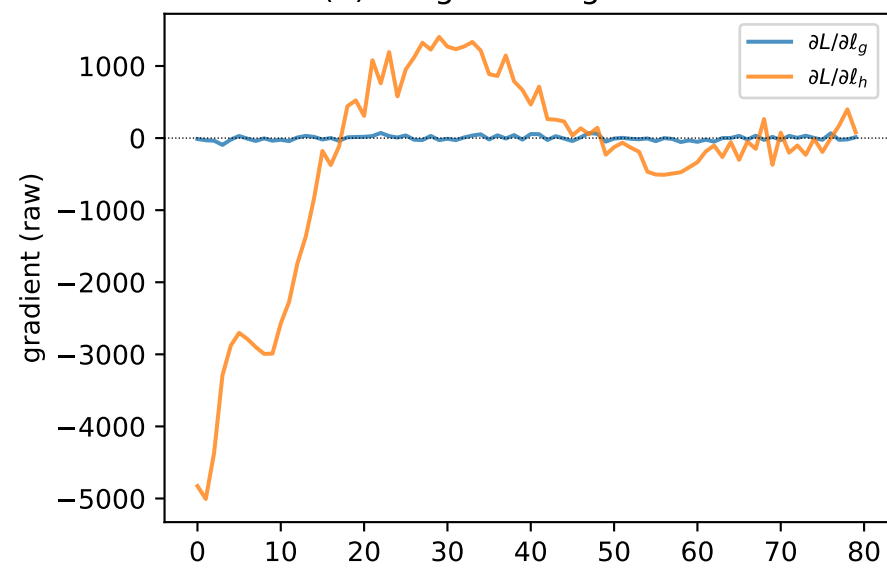
(d) Lengthscale gradients
