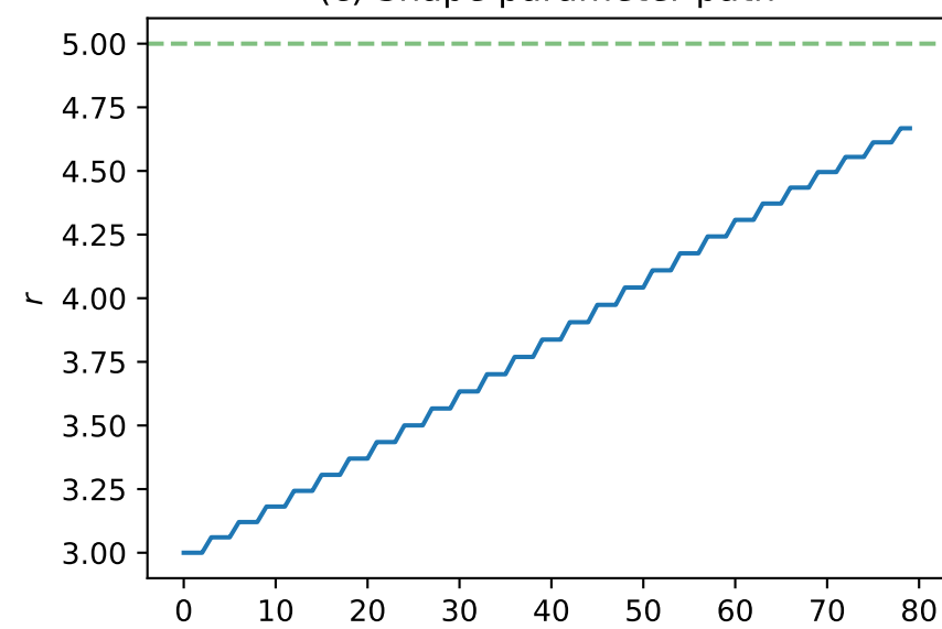
(c) Shape parameter path
