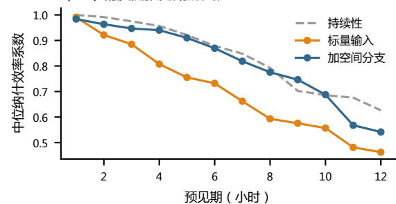
(乙) 精度随预见期的变化
