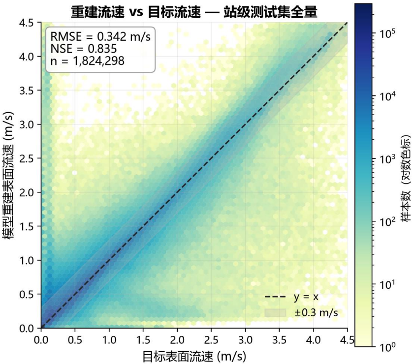
图1 纯净版重建流速 vs 目标流速密度图 (测试集全量182 万线, 对数色标)。主对角带紧密; 虚线y=x, 灰带 ±0.3 m/s。
