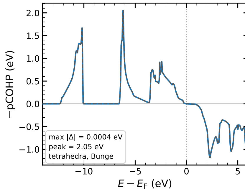
GaAs, Ga-As
