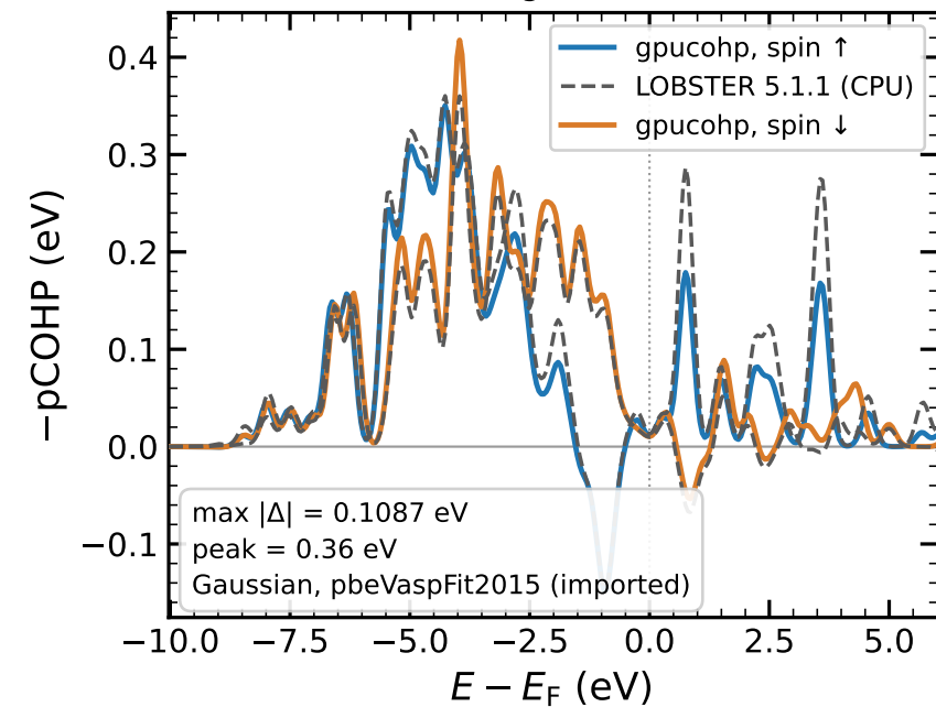
FeNi 3 , Fe-Ni
