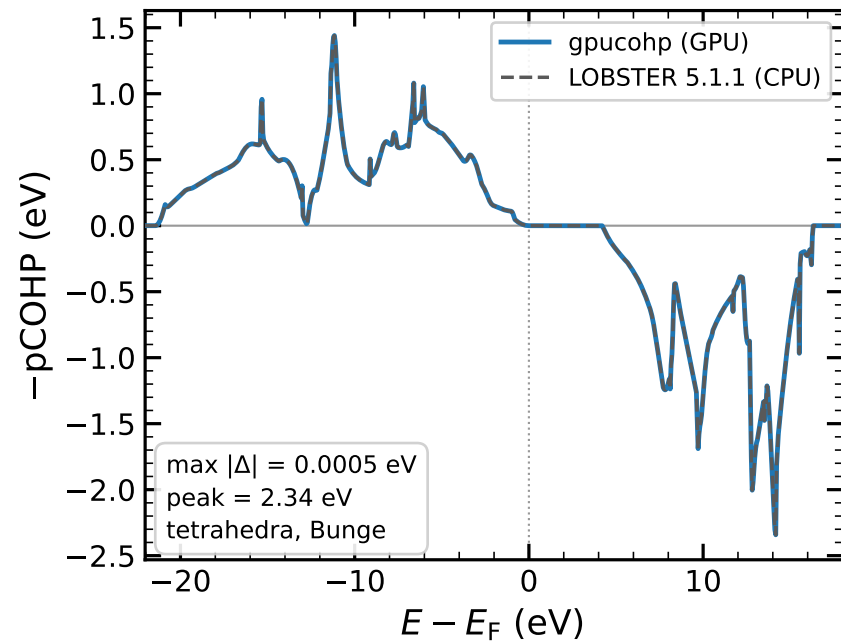
diamond, C-C
