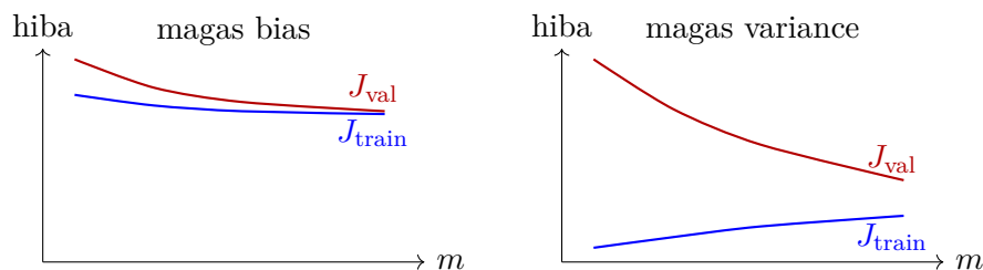
2. ábra. Tanulási görbék sematikusán: bias esetén a két hiba magas szinten összezár, variance esetén nagy a rés a tanító és validációs hiba között.
