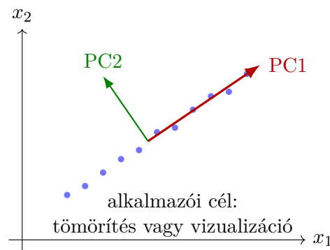
5. ábra. PCA alkalmazói szemléletben: nagy varianciájú irányokra vetítjük az adatot.
