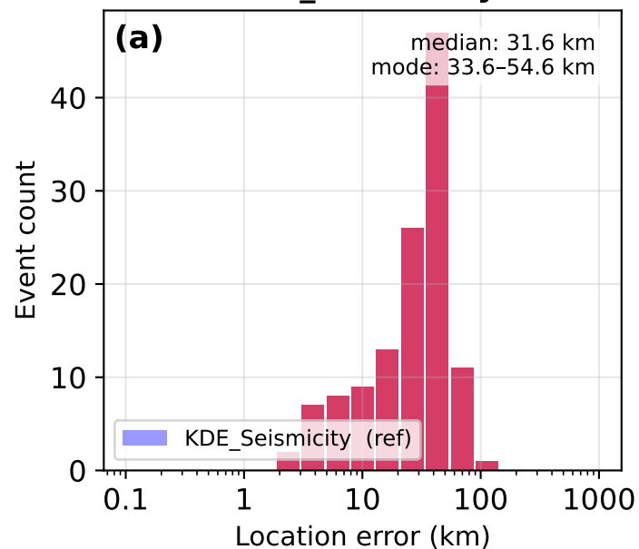
KDE_Seismicity
