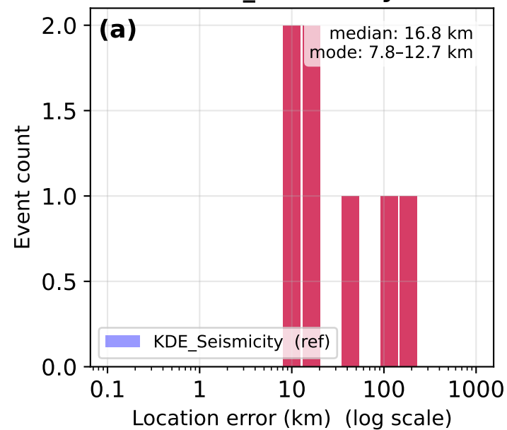
KDE_Seismicity
