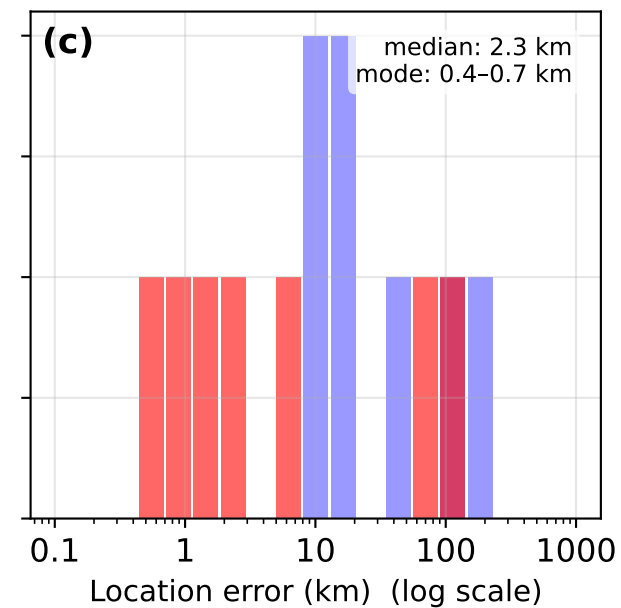
ETAS
