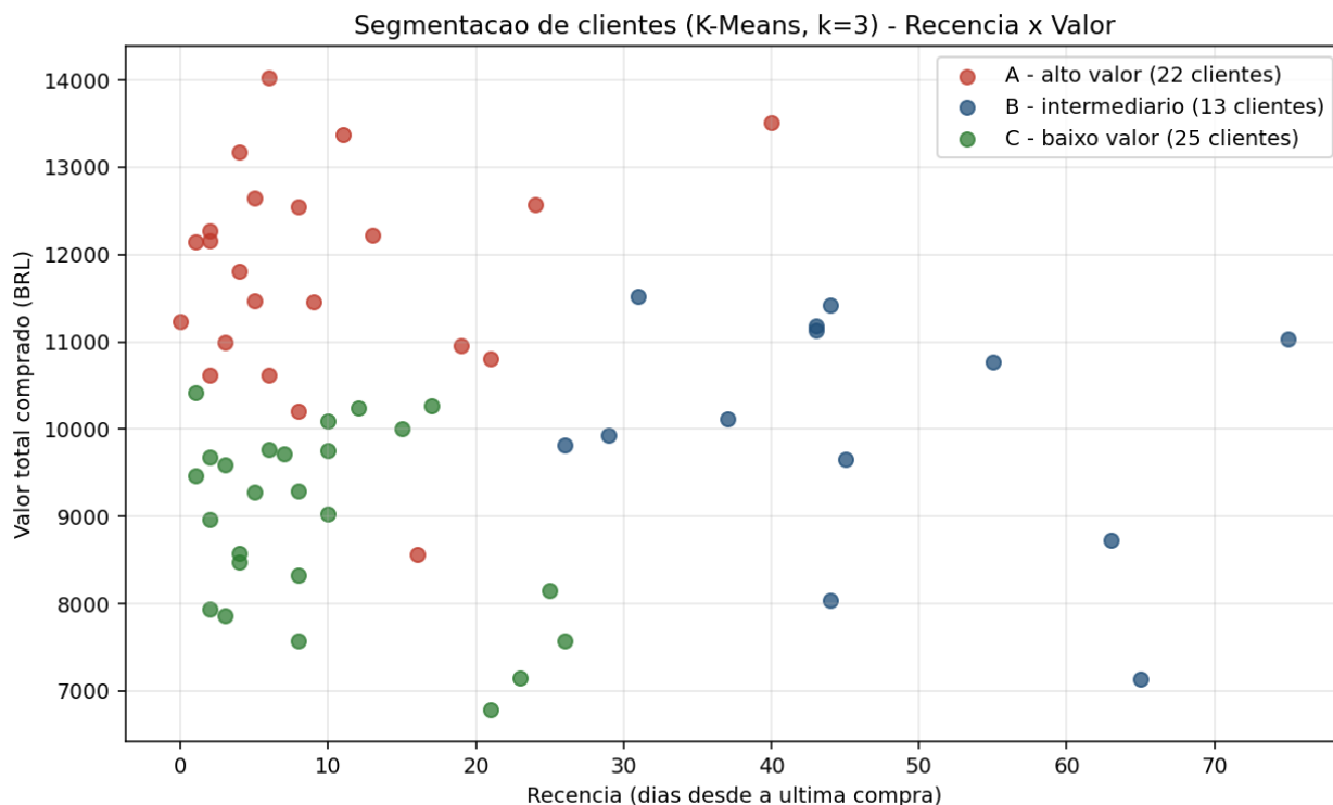
Figura 7 — Segmentação de clientes por K-Means ( k=3 ) sobre recência \times valor.
