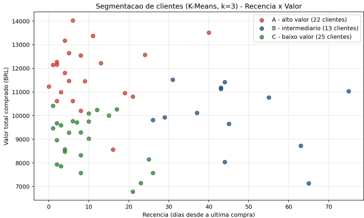
Figura 3 — Segmentação de clientes (K-Means, k=3) sobre recência x valor.
