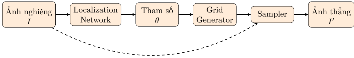
Hình 3.5: Kiến trúc Spatial Transformer Network
