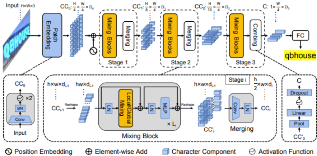
Hình 3.7: Kiến trúc tổng quan của SVTR (nguồn: Du et al., 2022)
