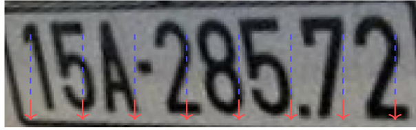
Ảnh biển số được chia thành các “lát cắt” dọc \downarrow mỗi lát \rightarrow vector đặc trưng D chiều
