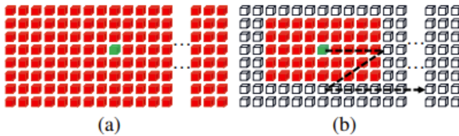
Hình 3.9: So sánh Local Mixing và Global Mixing trong SVTR
